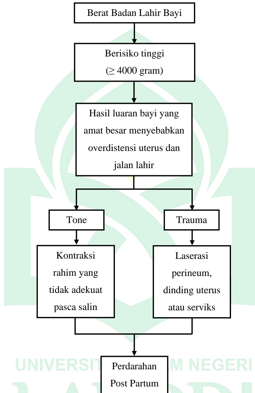
Gambar 2.1 Kerangka Teori
