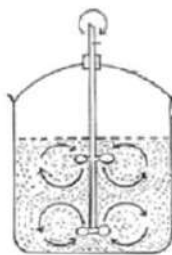
Gambar 2. Alat Maserasi Dengan Kelengkapan Pengaduk (Saputra, 2020)
