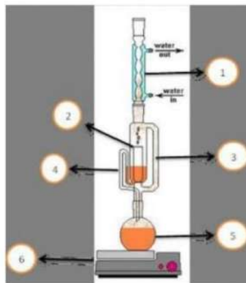
Gambar 4. Alat Soxhletasi (Saputra, 2020)
