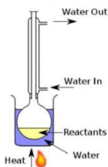
Gambar 3. Alat Refluks (Saputra, 2020)
