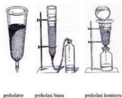
Gambar 5. Alat Proses Perkolasi (Saputra, 2020)
