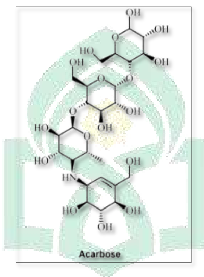
Gambar 7. Struktur Kimia Acarbose (Dirir et al., 2022)
