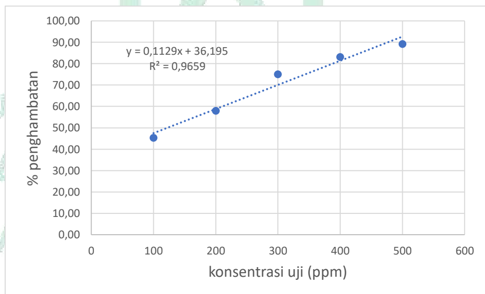
Gambar 10. Kurva fraksi etil asetat rimpang lempuyang gajah ( Zingiber zerumbet L.)
