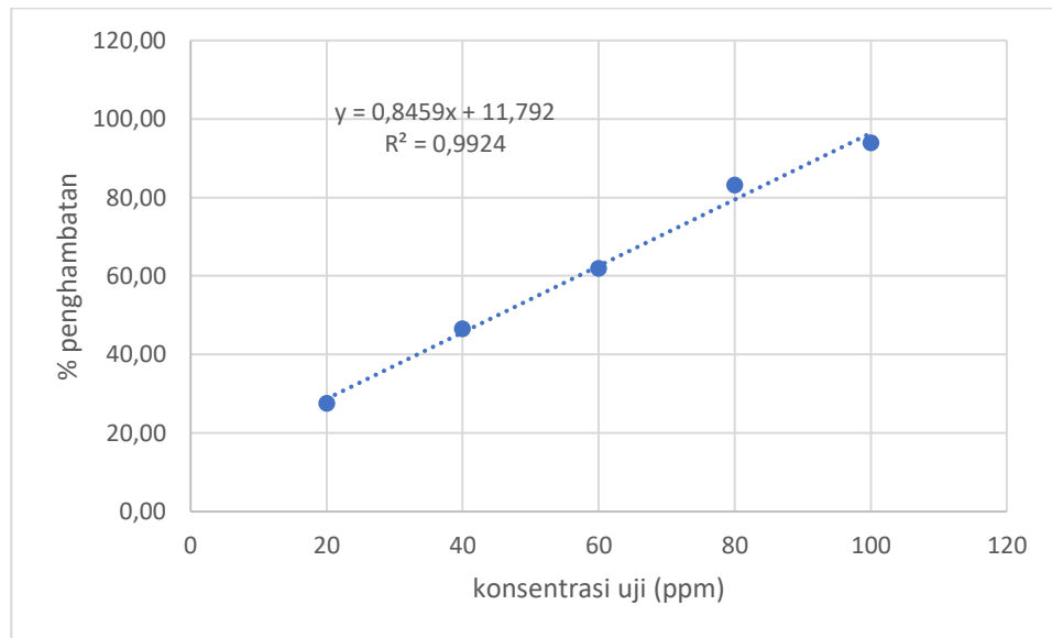
Gambar 11. Kurva kontrol positif acarbose
