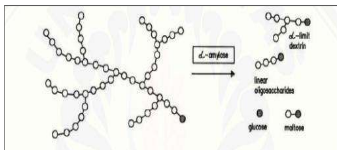
Gambar 5. Hidrolisis Pati oleh Enzim \alpha -amilase (Timerman, 2012)
