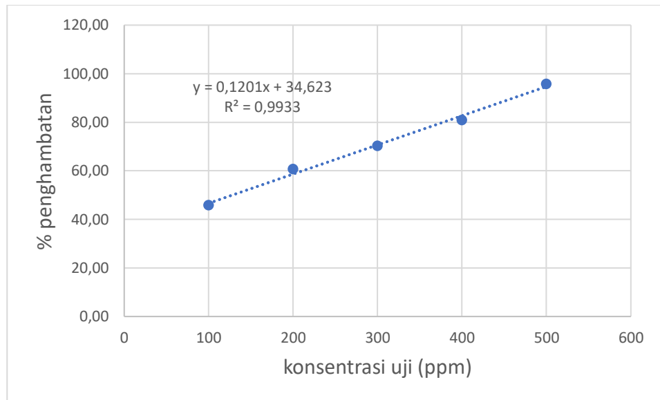
Gambar 9. Kurva fraksi n-heksan rimpang lempuyang gajah ( Zingiber zerumbet L.)
