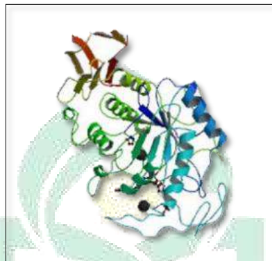
Gambar 4. Struktur enzim \alpha -amilase (Sundarram & Murthy, 2014)
