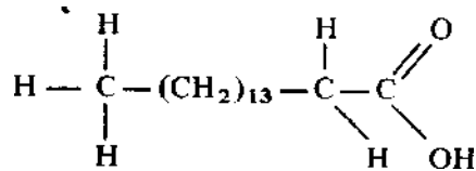
Gambar 2.1 Struktur Kimia Asam Lemak (Almatsier, 2016).
