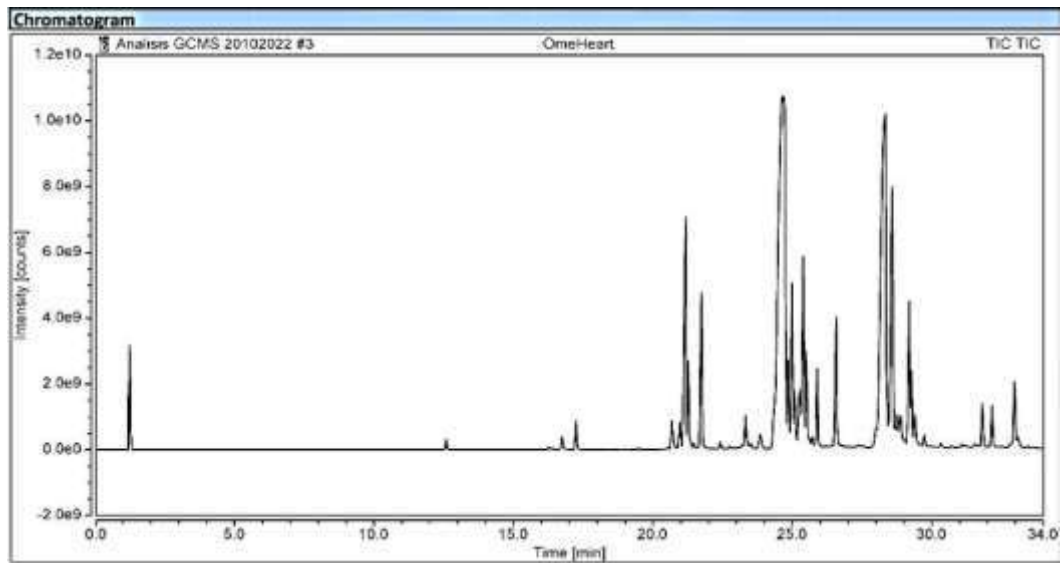
Kromatogram sampel C
