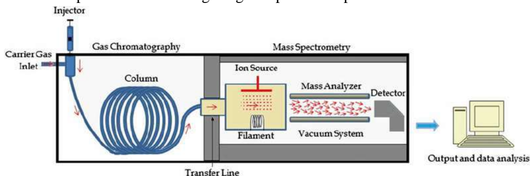
Gambar 3. Skema Alat Kromatografi Gas
