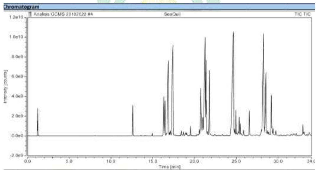
Kromatogram sampel D
