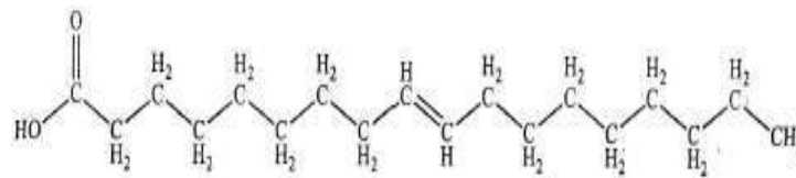
Gambar 2.3 Struktur Asam Lemak Tak Jenuh Tunggal ( Mono Unsaturated Fatty Acid ) (Almatsier, 2016).
