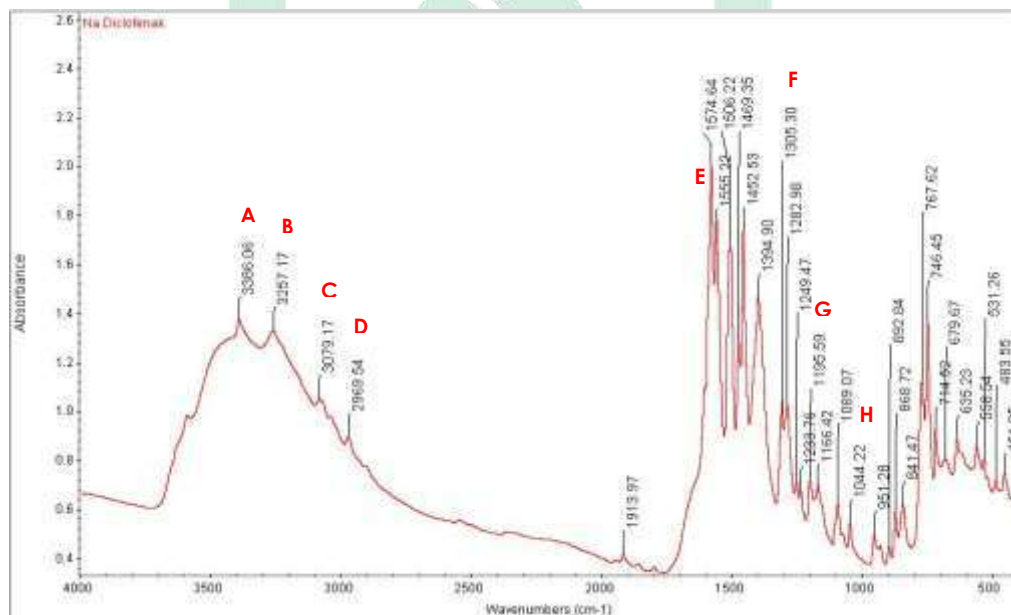
Gambar 4. Spektrum Standar Natrium Diklofenak
