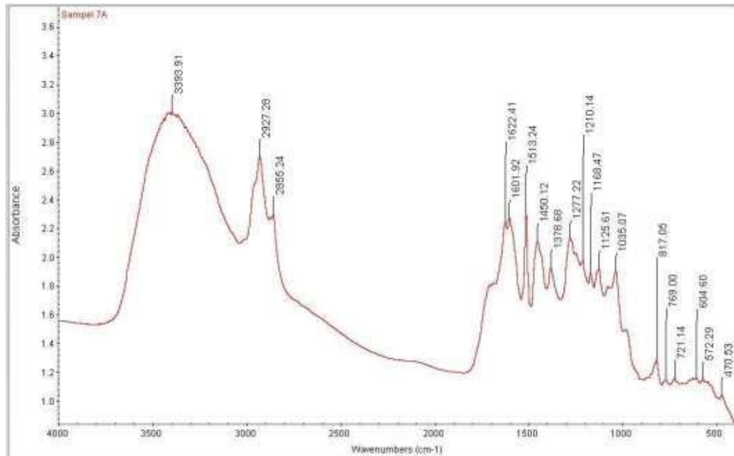
Gambar 53. Spektrum Jamu Pegal Linu JSR A
