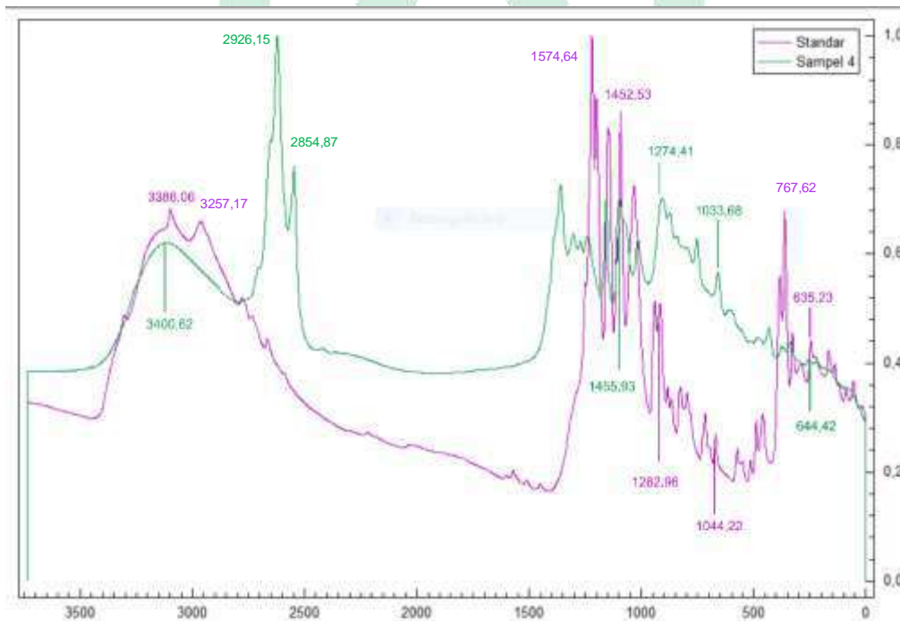
Gambar 8. Spektrum Standar Natrium Diklofenak dengan Sampel 4 Jamu Pegal Linu-Rat Cap Sido Mekar
