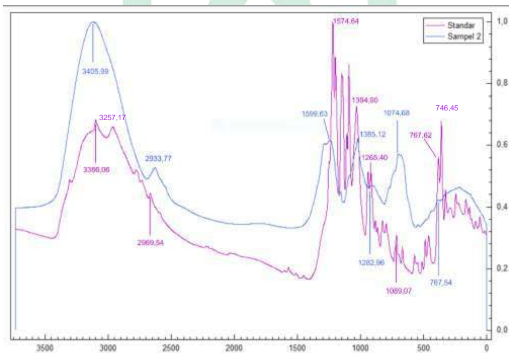
Gambar 6. Spektrum Standar Natrium Diklofenak dengan Sampel 2 Jamu Pegal Linu Cap Sinar Serambi
