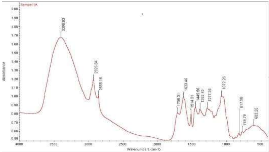
Gambar 35. Spektrum Jamu Sabdo Palon
