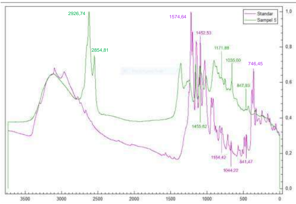
Gambar 9. Spektrum Standar Natrium Diklofenak dengan Sampel 5 Jamu Pegal Linu Plus Ginseng
