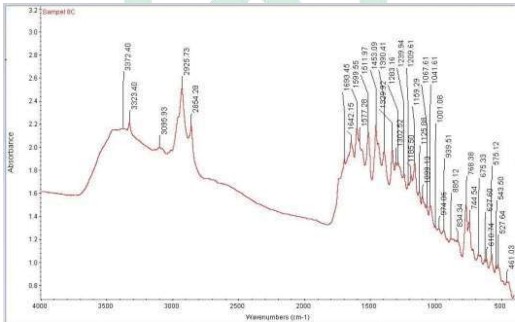
Gambar 58. Spektrum Jamu Pegal Linu Cap Bunga Matahari C
