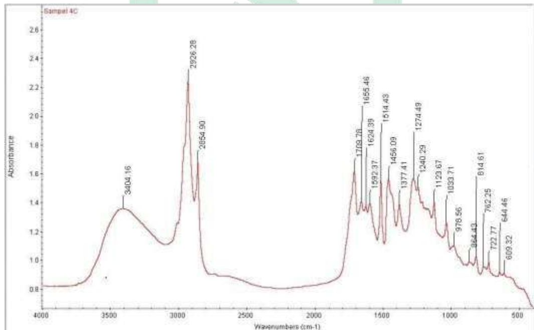
Gambar 46. Spektrum Jamu Pegal Linu-Rat C
