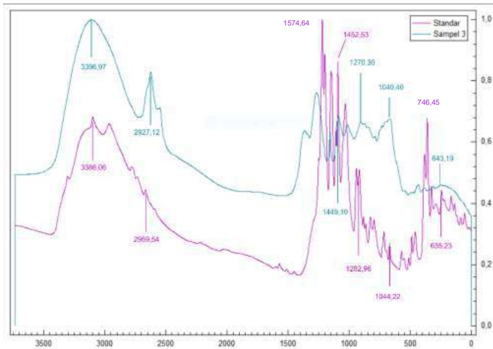
Gambar 7. Spektrum Standar Natrium Diklofenak dengan Sampel 3 Jamu Pegal Linu 10
