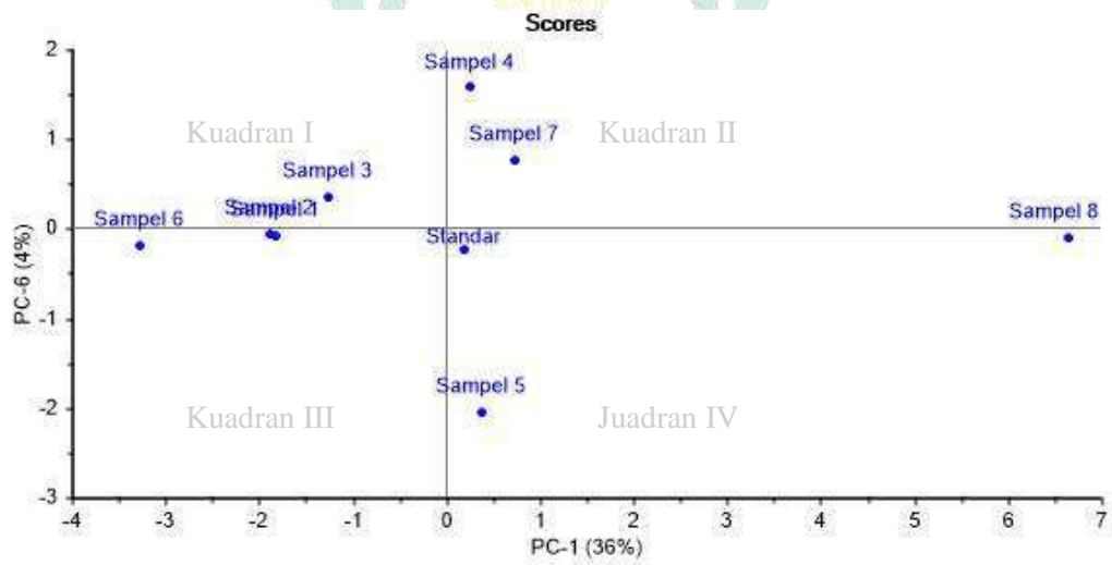
Gambar 63. Score Plot PCA PC-1 dan PC-6
