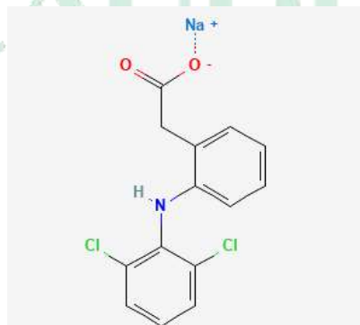
Gambar 2. Struktur Natrium Diklofenak (NCBI, 2022).
