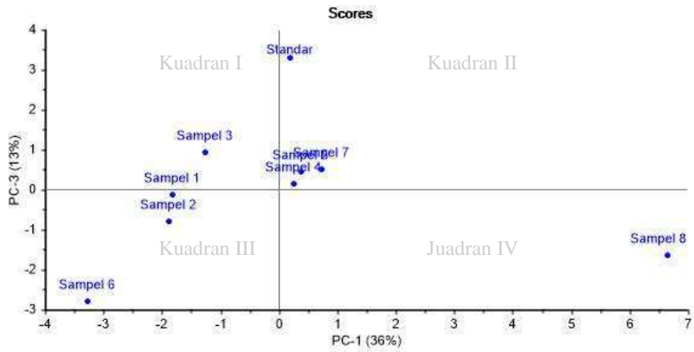
Gambar 60. Score Plot PCA PC-1 dan PC-3
