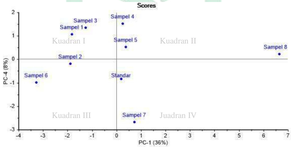
Gambar 61. Score Plot PCA PC-1 dan PC-4
