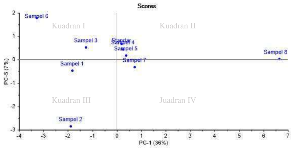
Gambar 62. Score Plot PCA PC-1 dan PC-5
