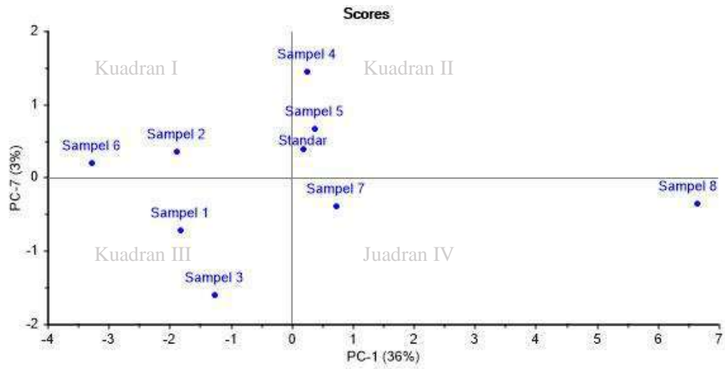
Gambar 64. Score Plot PCA PC-1 dan PC-7
