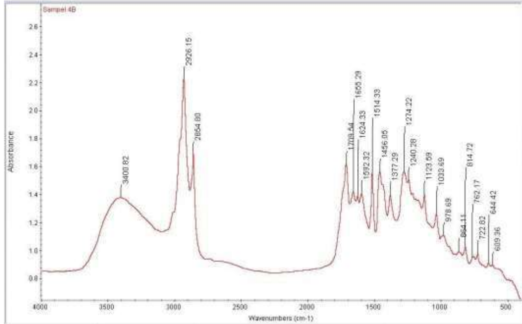
Gambar 45. Spektrum Jamu Pegal Linu-Rat B
