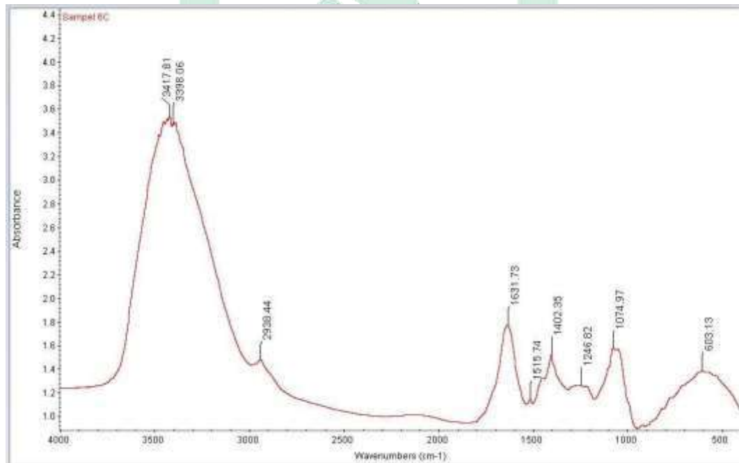
Gambar 52. Spektrum Jamu Pegal Linu Lengkap C
