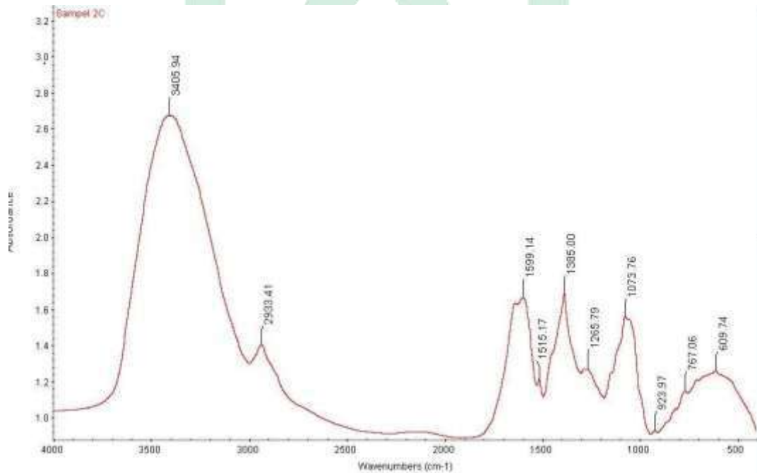
Gambar 40. Spektrum Jamu Pegal Linu Reumatik Sinar Serampi C
