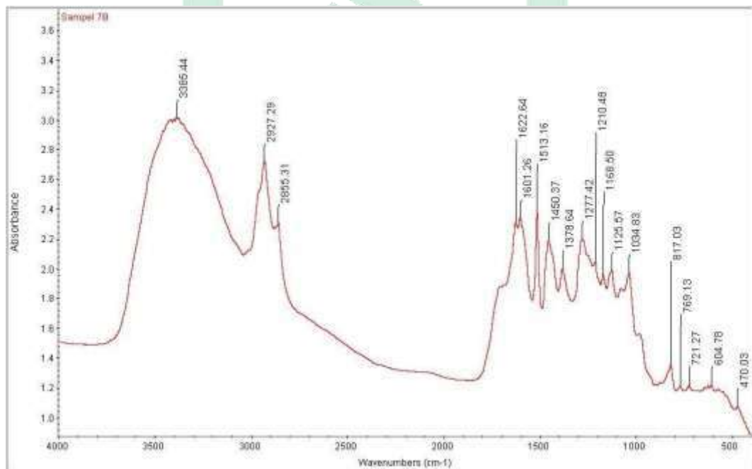
Gambar 54. Spektrum Jamu Pegal Linu JSR B
