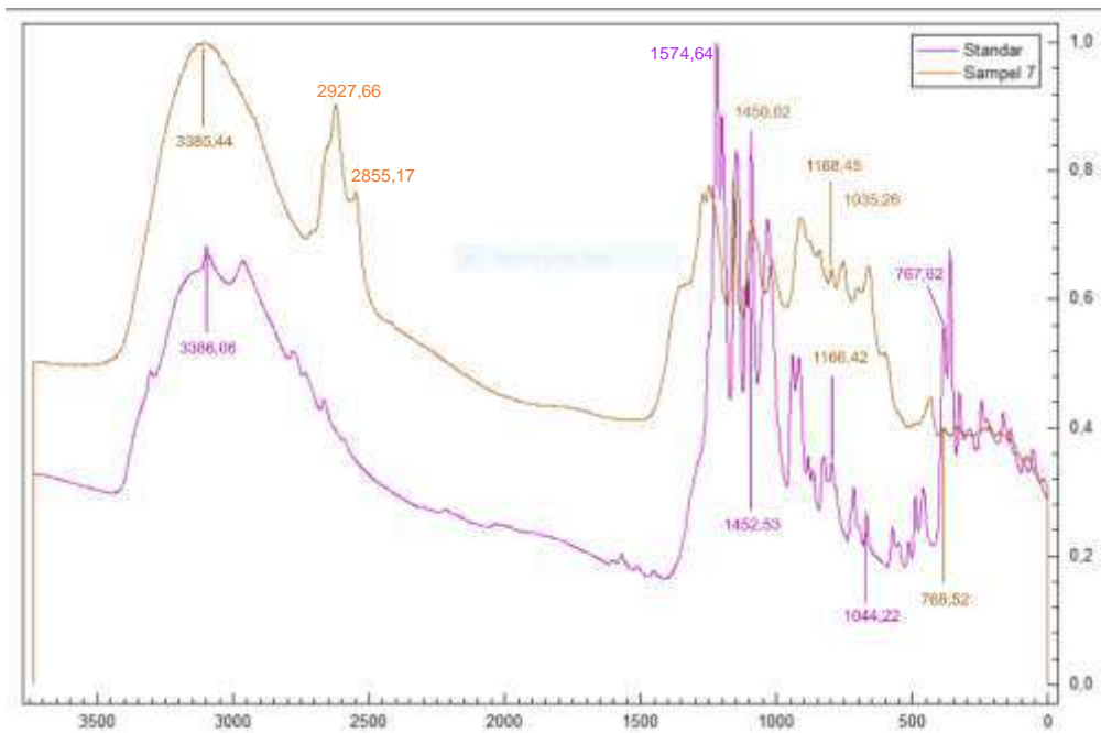
Gambar 11. Spektrum Standar Natrium Diklofenak dengan Sampel 7 Jamu Pegal Linu JSR
