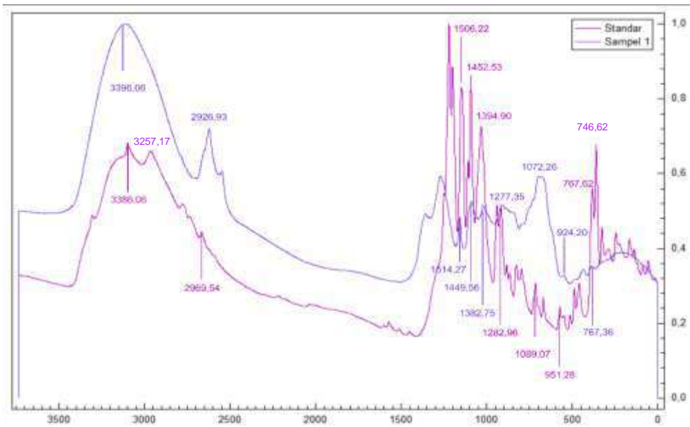
Gambar 5. Spektrum Standar Natrium Diklofenak dengan Sampel 1 Jamu Pegal Linu Sabdo Palom
