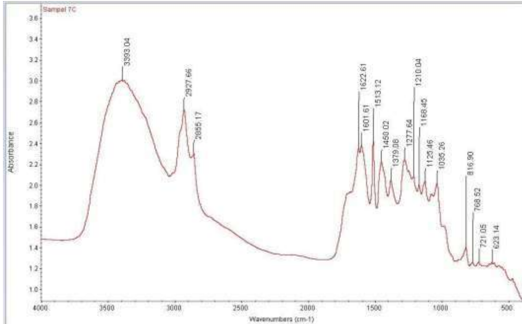
Gambar 55. Spektrum Jamu Pegal Linu JSR C
