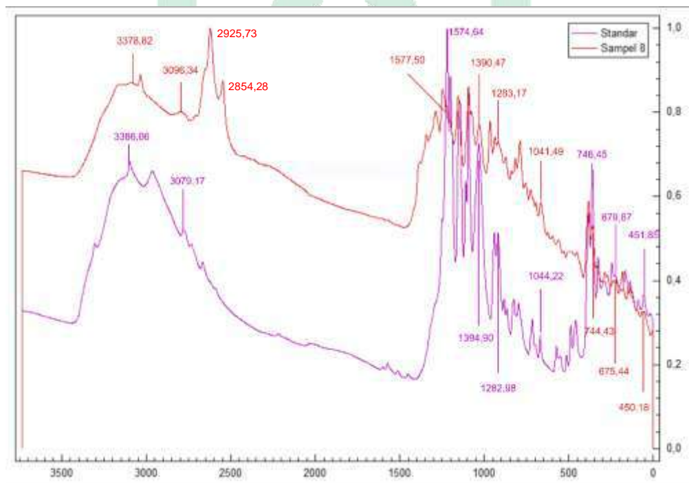
Gambar 12. Spektrum Standar Natrium Diklofenak dengan Sampel 8 Jamu Pegal Linu Cap Bunga Matahari
