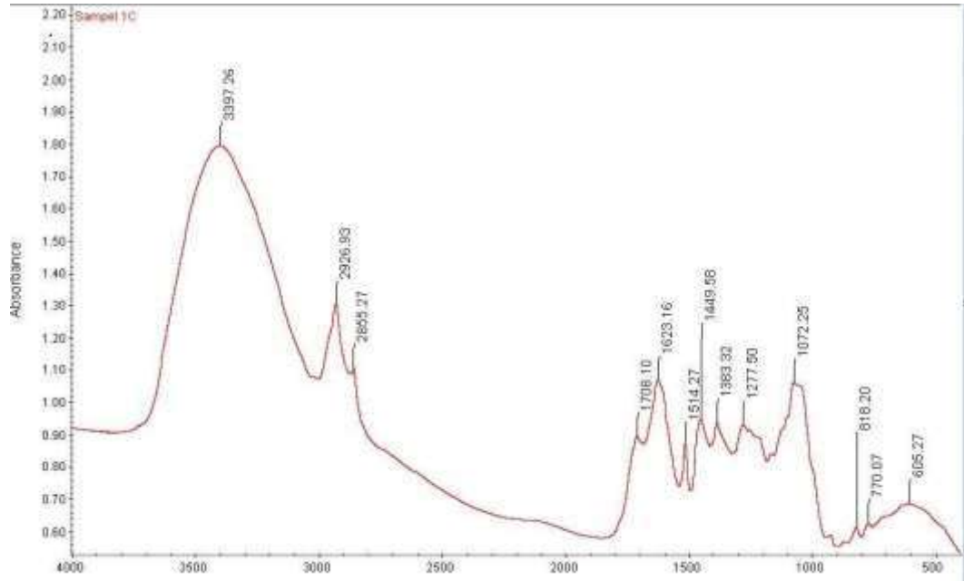
Gambar 37. Spektrum Jamu Sabdo Palon C
