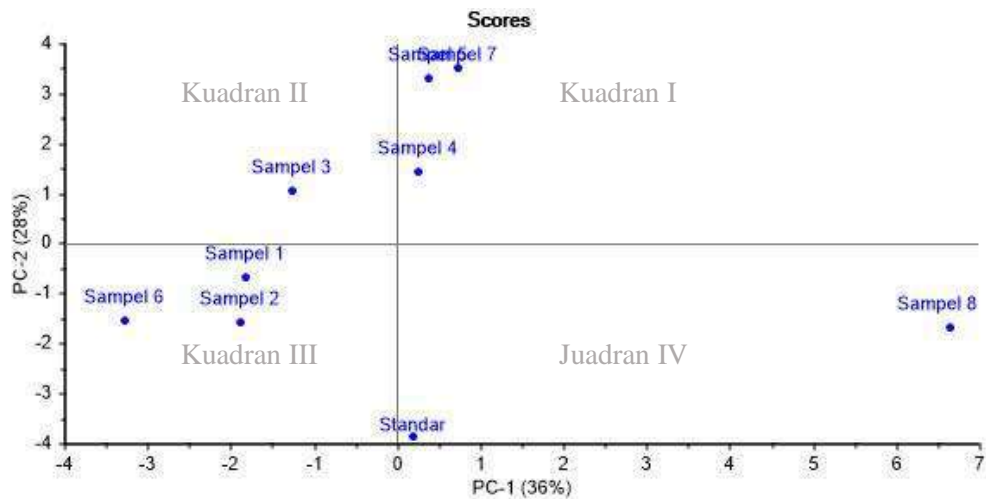
Gambar 13. Score Plot PCA PC-1 dan PC-2
