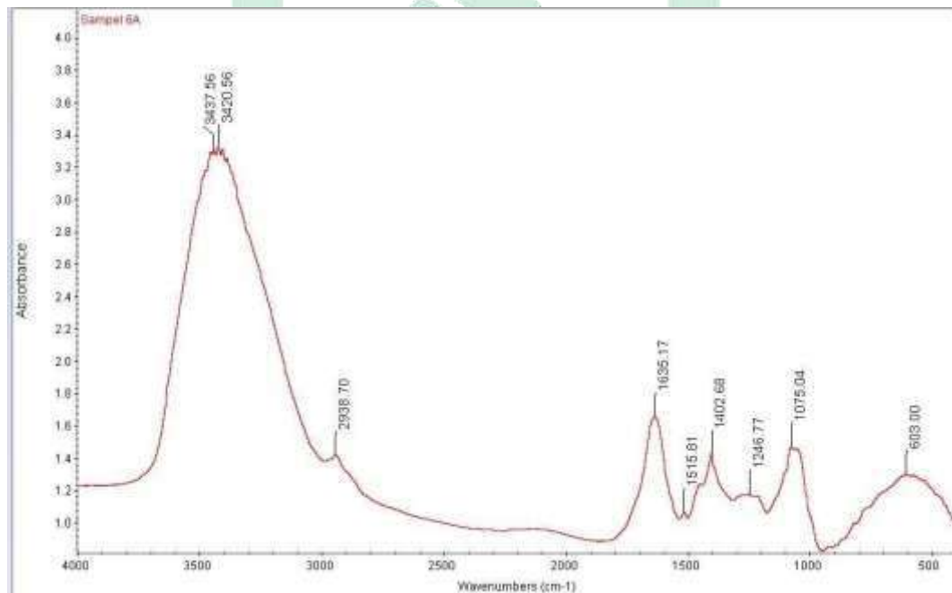
Gambar 50. Spektrum Jamu Pegal Linu Lengkap A
