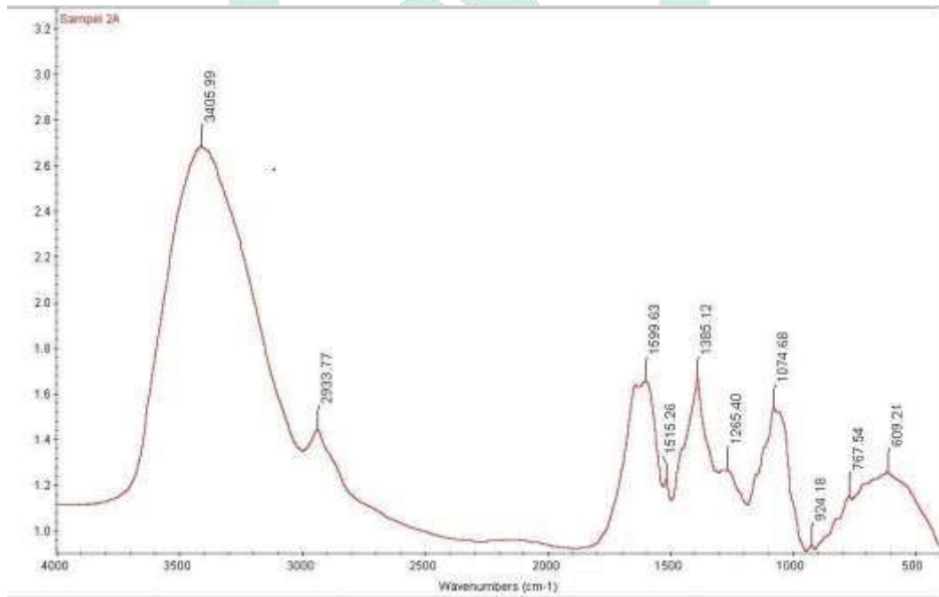
Gambar 38. Spektrum Jamu Pegal Linu Reumatik Sinar Serampi A
