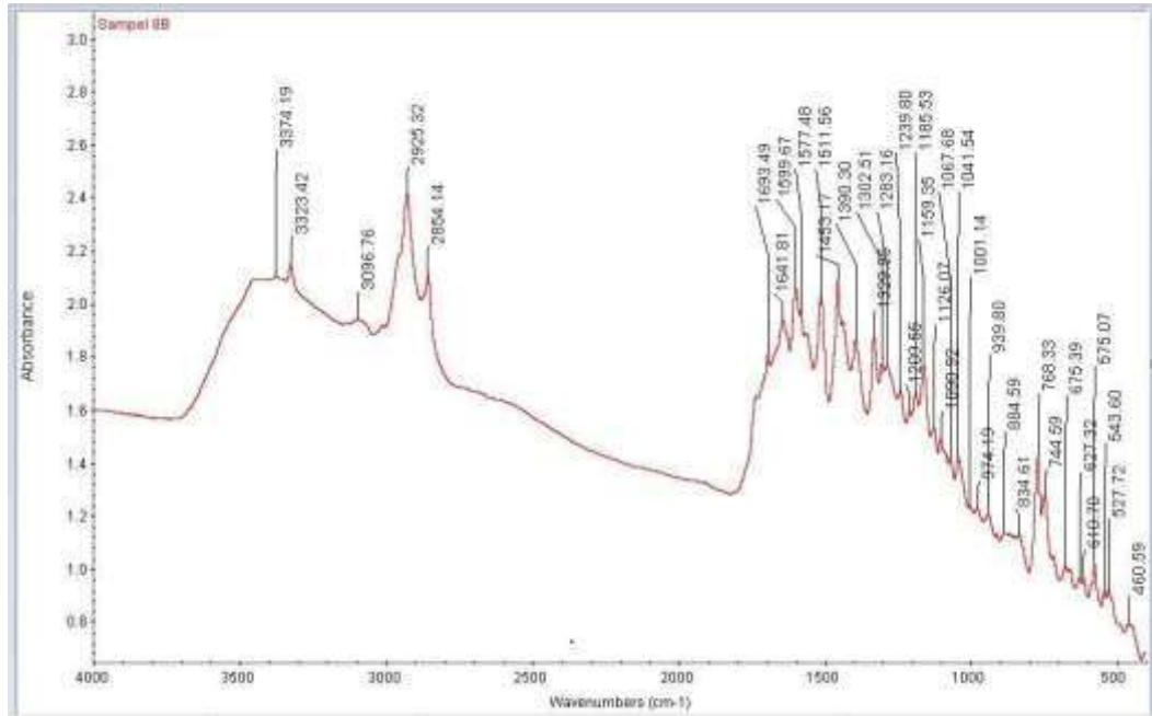
Gambar 57. Spektrum Jamu Pegal Linu Cap Bunga Matahari B
