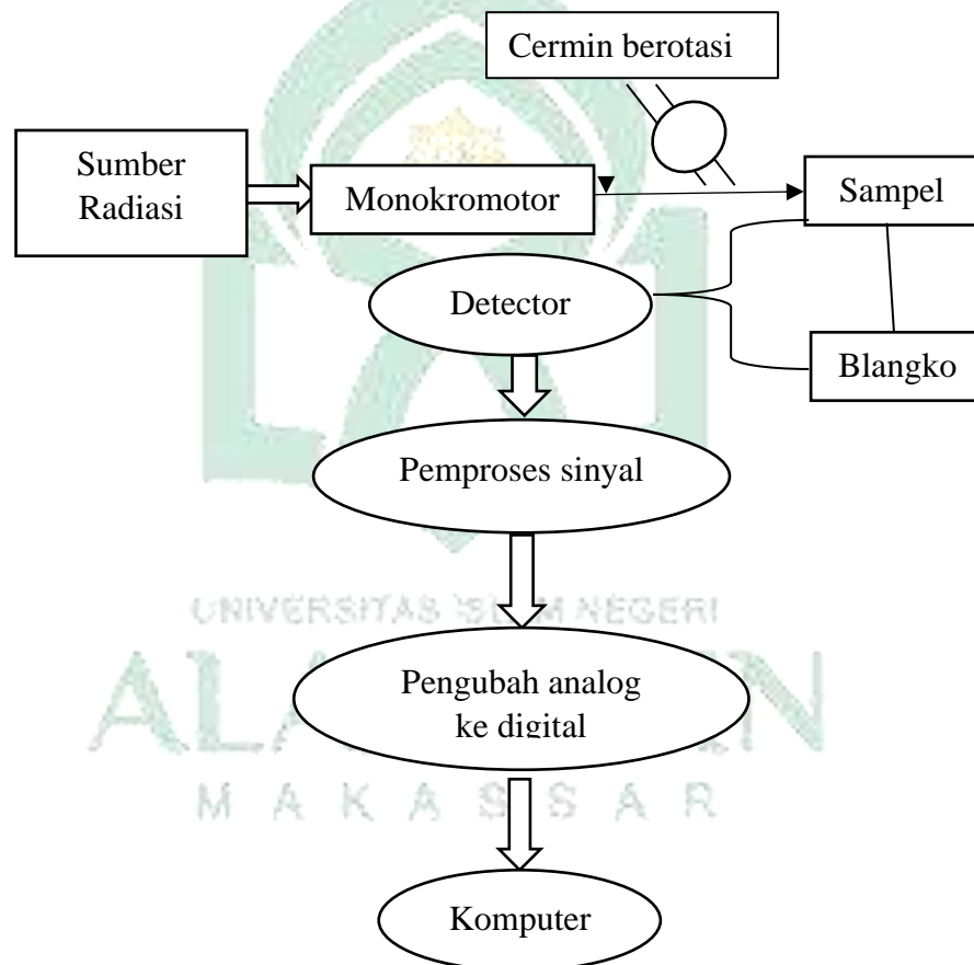
(Gambar 2 6 Skema Kerja Spektrofotometri UV-Vis (Mulja, 1995))
