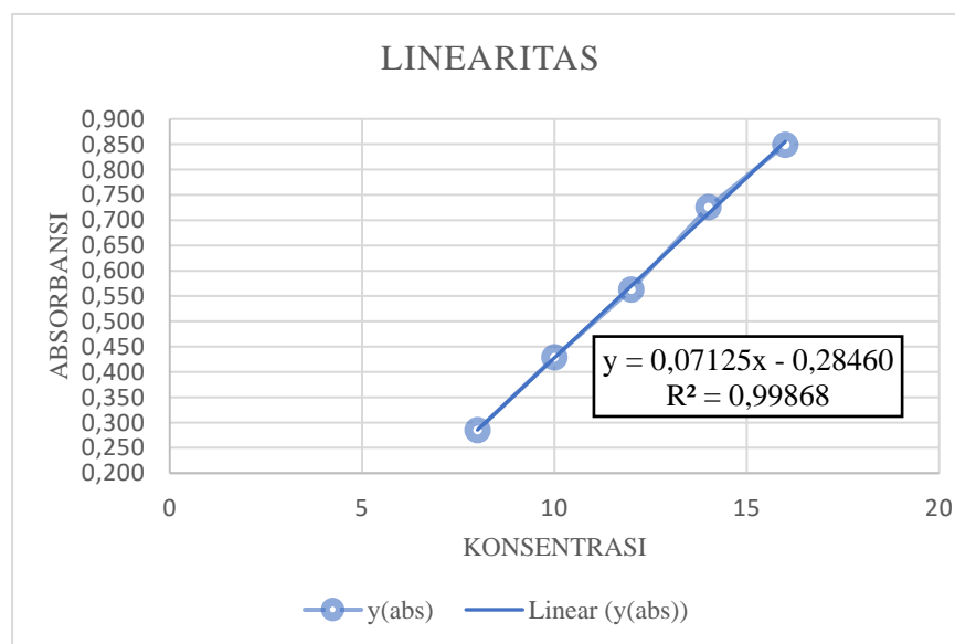
Gambar 4.1 (Kurva Larutan Baku Linearitas)
