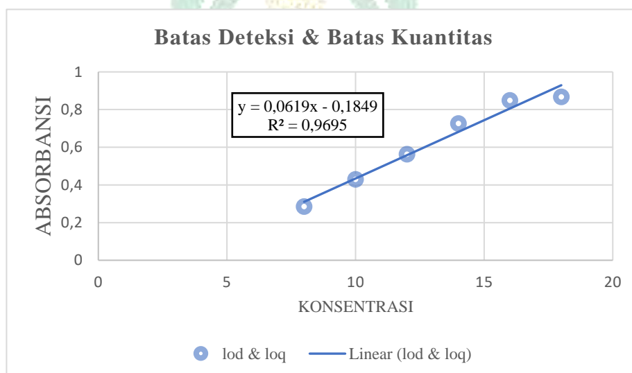
Gambar 4.2 (Kurva kalibrasi penentuan batas deteksi dan batas kuantitas)
