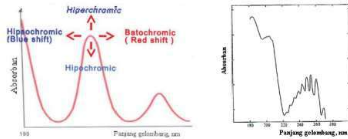
(Gambar 2 4 Gambaran Spektrum UV-Vis)
