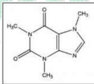
(Gambar 2 1 Struktur Kimia Kafein)
