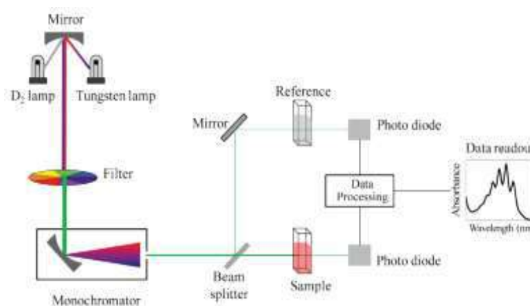
(Gambar 2.3 Skema Spektrofotometer UV-vis Double Beam )
