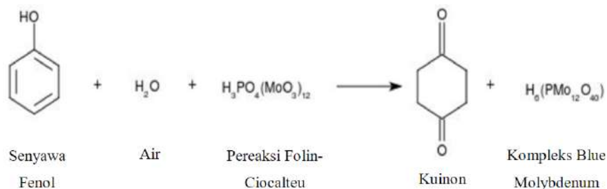
Gambar 2. Reaksi senyawa fenolik dengan reagen Folin-Ciocalteu (Noviyanty, Hepiyansoro, & Agustian, 2020).
