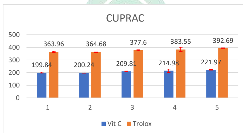
Gambar 13. Diagram kapasitas antioksidan CUPRAC
