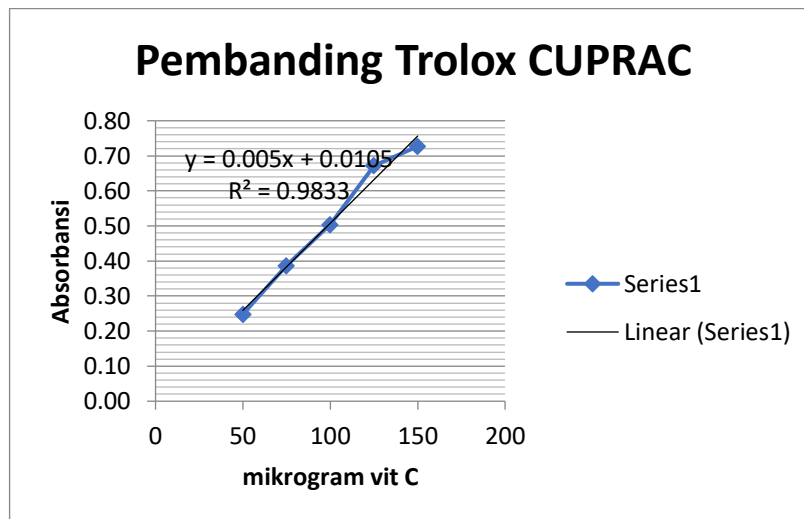
Gambar 20. Kurva baku trolox metode CUPRAC
