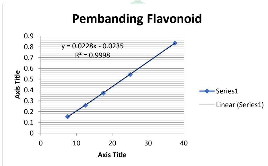
Gambar 16. Kurva baku kuersetin
