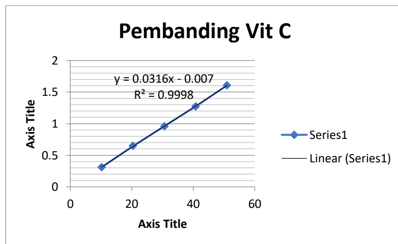
Gambar 23. Kurva baku asam askorbat metode TOAC
