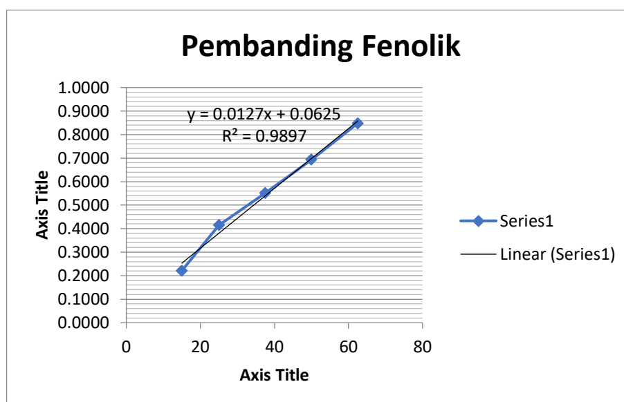
Gambar 15. Kurva baku asam galat
