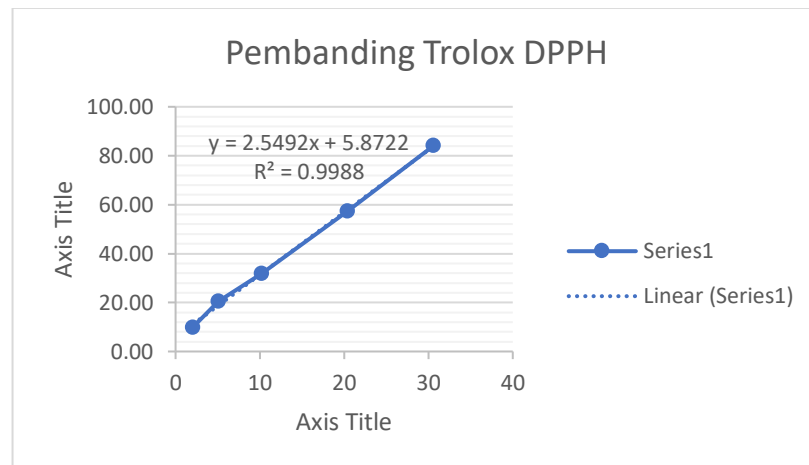
Gambar 22. Kurva baku trolox metode DPPH
