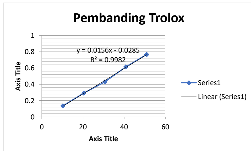
Gambar 24. Kurva baku trolox metode TOAC
