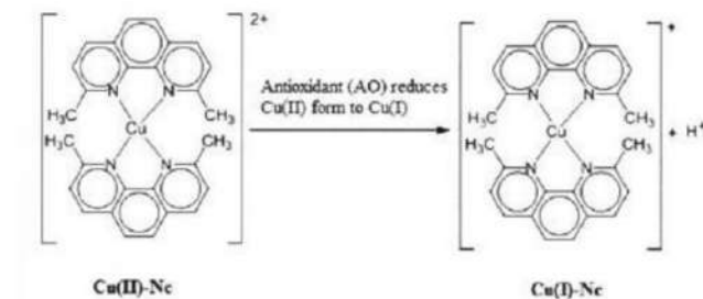
Gambar 12. Reaksi metode CUPRAC
