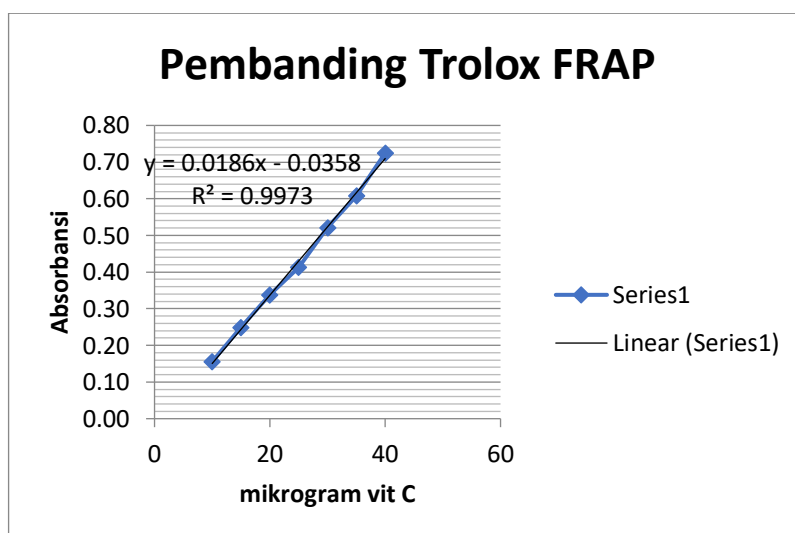
Gambar 18. Kurva baku trolox metode FRAP
