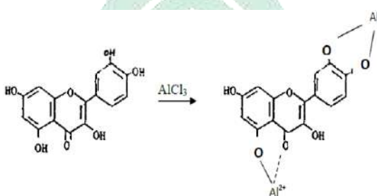
Gambar 4. Pembentukan senyawa kompleks kuersetin-aluminium klorida
