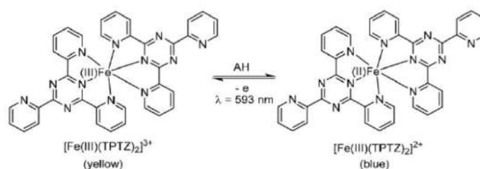
Gambar 10. Reaksi metode FRAP
