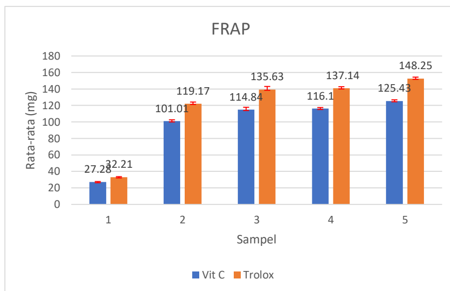
Gambar 11. Grafik kapasitas antioksidan FRAP
