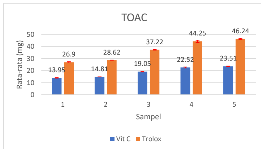
Gambar 7. Diagram Kapasitas Antioksidan TOAC
