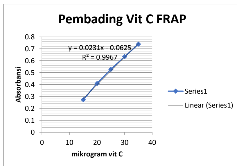
Gambar 17. Kurva baku asam askorbat metode FRAP
