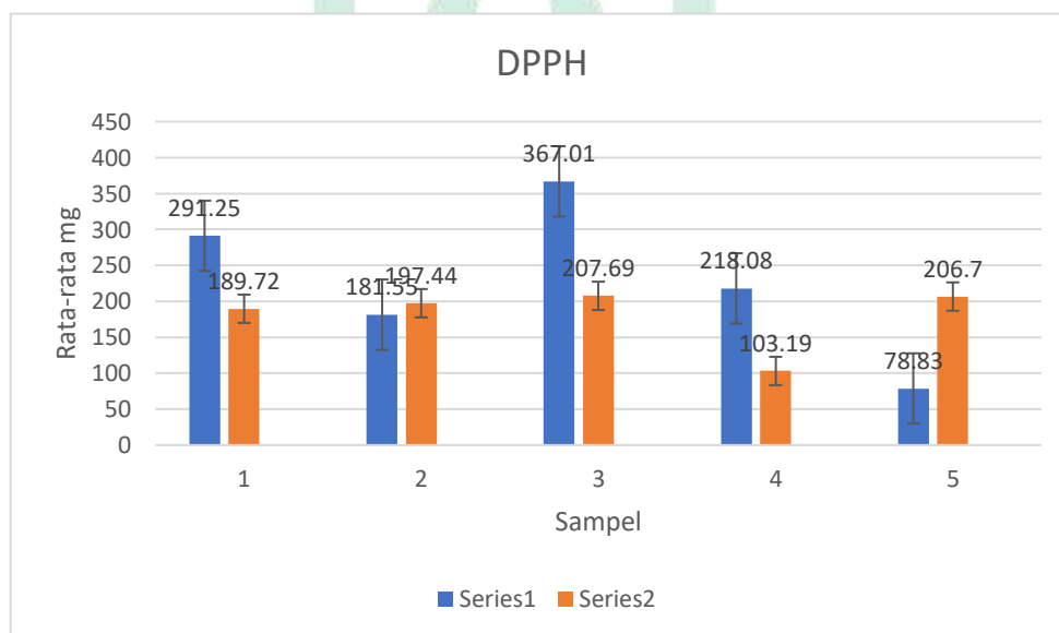
Gambar 9. Diagram Kapasitas Antioksidan DPPH
