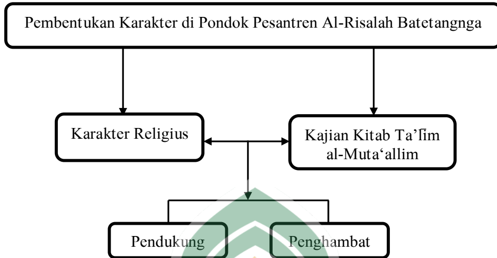
Gambar 2.1 Kerangka Teoretis
