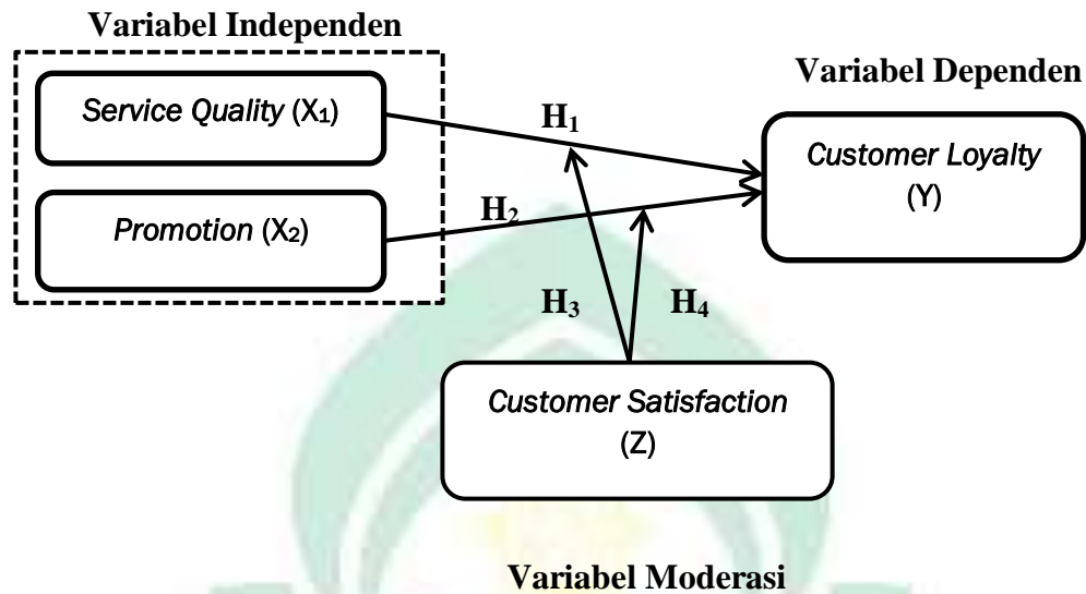
Gambar 2.1 Kerangka Pemikiran
