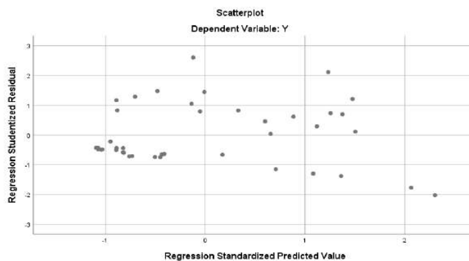
Gambar 4.2 Uji Heteroskedastisitas
