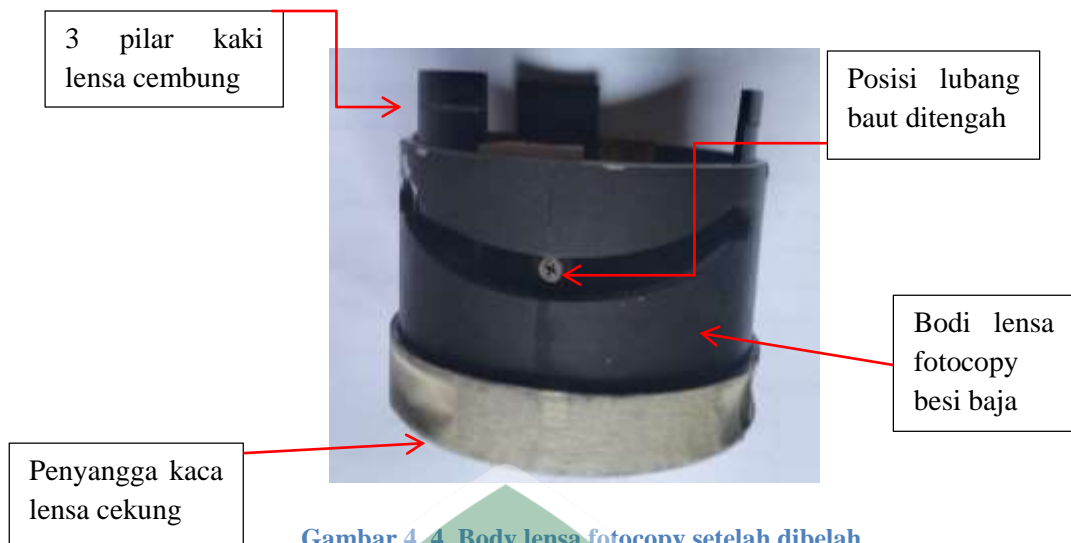
Gambar 4. 4. Body lensa fotocopy setelah dibelah
