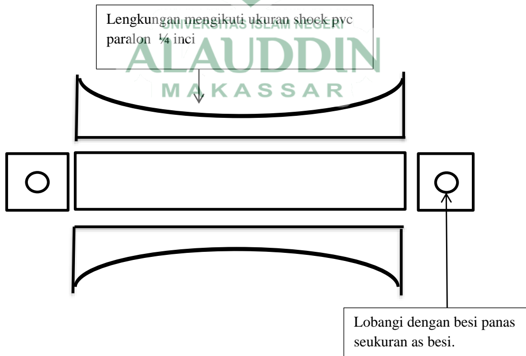
Gambar 4. 13. Potongan lembaran pvc
