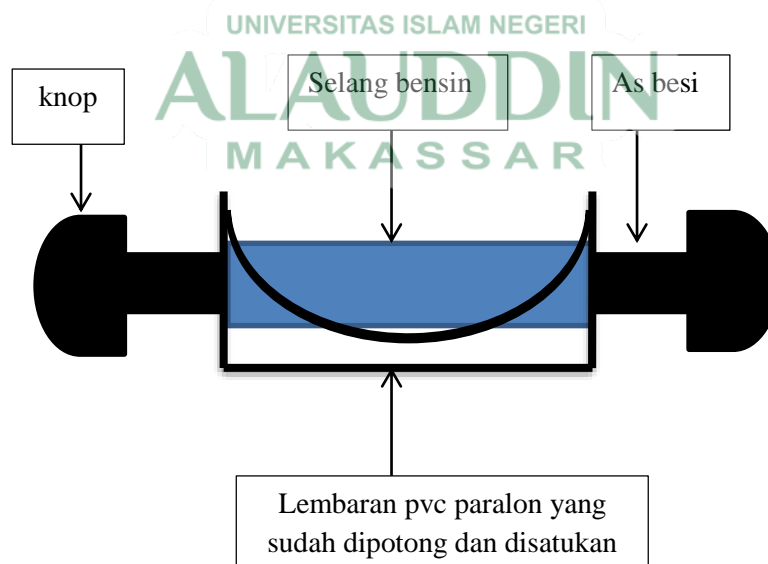
Gambar 4. 17. Skema letak posisi pengatur fokuser
