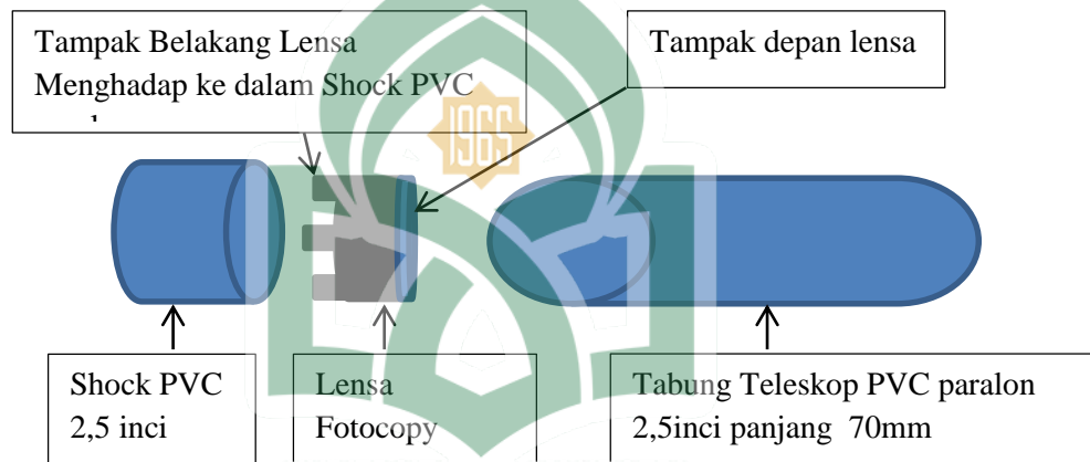
Gambar 4. 6. Skema posisi shock pvc, lensa dan body.
