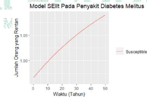
Gambar 4. 10 Penyebaran Jumlah Susceptible pada Penyakit Diabetes Melitus dengan Metode Runge Kutta Orde 4
