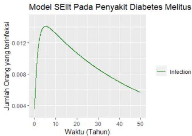
Gambar 4. 12 Penyebaran Jumlah Infection pada Penyakit Diabetes Melitus dengan Metode Runge Kutta Orde 4
