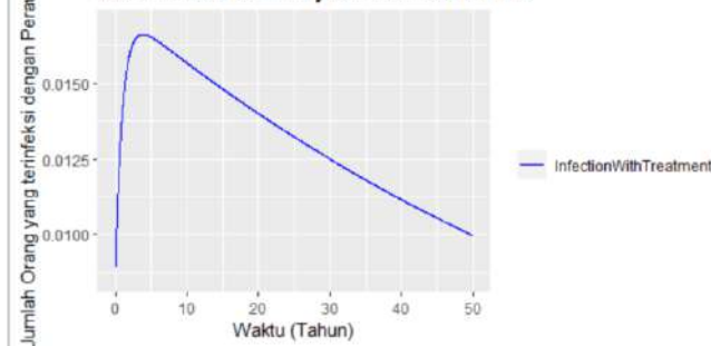
Model SEIIt Pada Penyakit Diabetes Melitus
