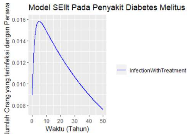
Gambar 4.13 Penyebaran Jumlah Infection With Treatment Penyakit Diabetes Melitus dengan Metode Runge Kutta Orde 4
