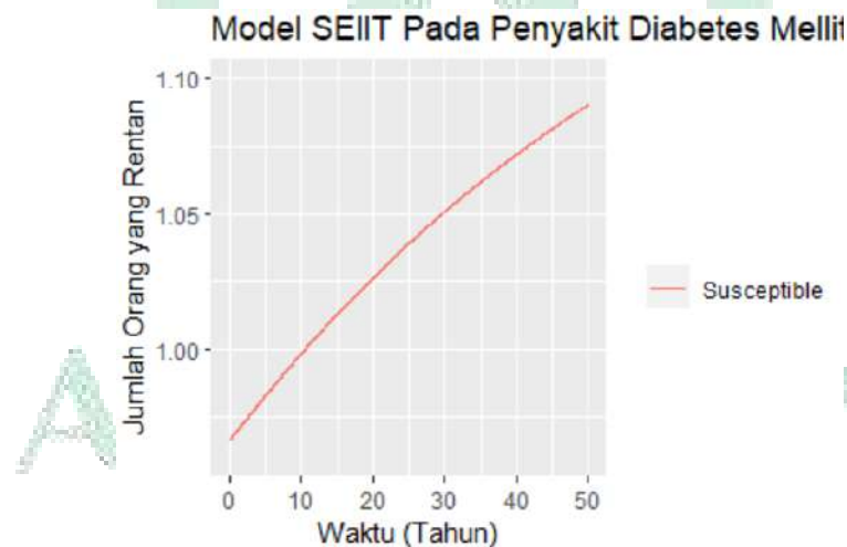
Gambar 4. 2 Penyebaran Jumlah Susceptible pada Penyakit Diabetes Melitus dengan Metode Euler
