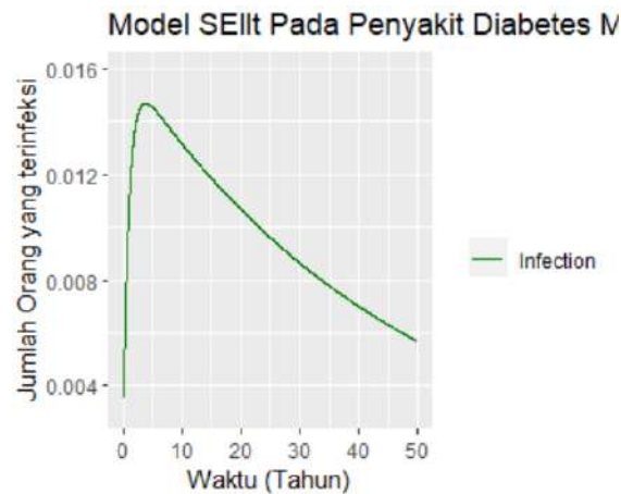
Gambar 4. 8 Penyebaran Jumlah Infection pada Penyakit Diabetes Melitus dengan Metode Heun
