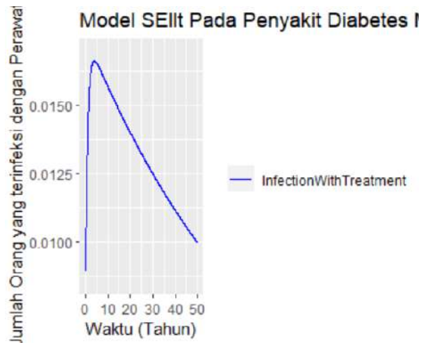
Gambar 4. 9 Penyebaran Jumlah Infection With Treatment Penyakit Diabetes Melitus dengan Metode Heun
