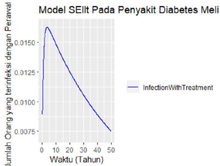
Gambar 4. 5 Penyebaran Jumlah Infection With Treatment Penyakit Diabetes Melitus dengan Metode Euler
