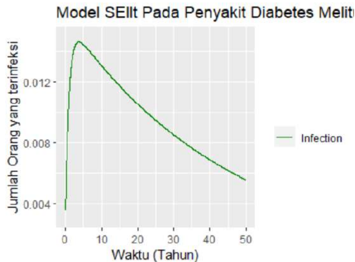
Gambar 4. 4 Penyebaran Jumlah Infection pada Penyakit Diabetes Melitus dengan Metode Euler
