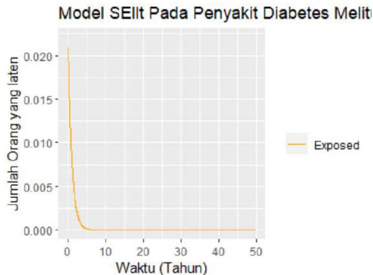
Gambar 4. 3 Penyebaran Jumlah Exposed pada Penyakit Diabetes Melitus dengan Metode Euler
