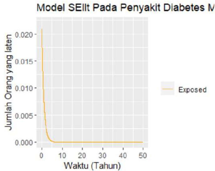
Gambar 4. 7 Penyebaran Jumlah Exposed pada Penyakit Diabetes Melitus dengan Metode Heun
