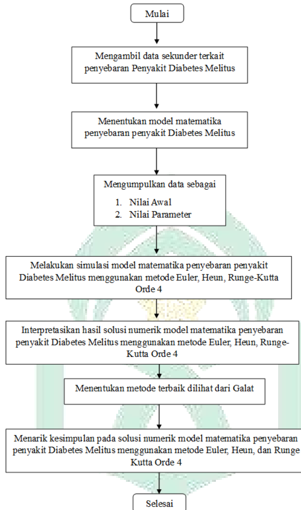
Gambar 3. 1 Skema Penyelesaian Masalah
