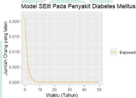
Gambar 4. 11 Penyebaran Jumlah Exposed pada Penyakit Diabetes Melitus dengan Metode Runge Kutta Orde 4
