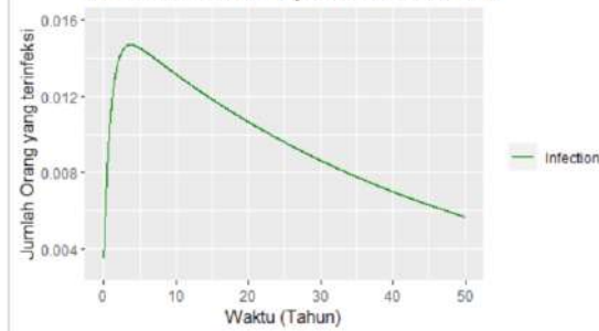
Model SEIIt Pada Penyakit Diabetes Melitus
