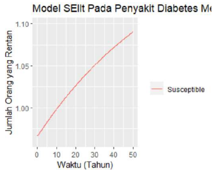
Gambar 4. 6 Penyebaran Jumlah Susceptible pada penyakit Diabetes Melitus dengan metode Heun
