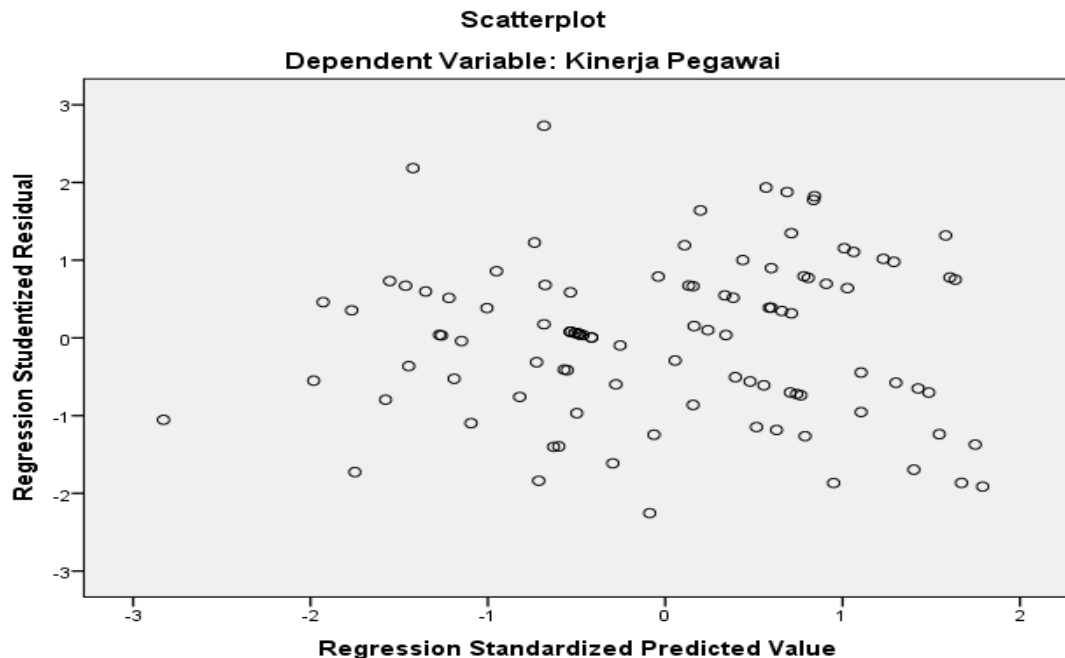
Gambar 4.1 Uji Heteroskedastisitas
