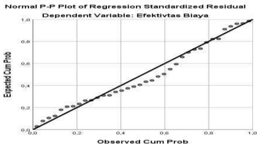
Gambar 4.2 Grafik P-P Plot
