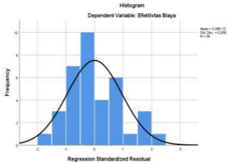
Gambar 4.1 Grafik Histogram
