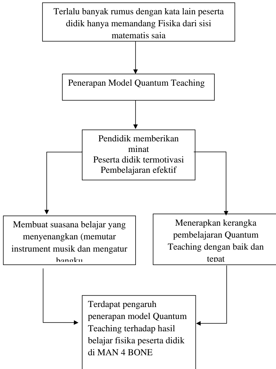
Gambar 2. 4 Kerangka Pikir
