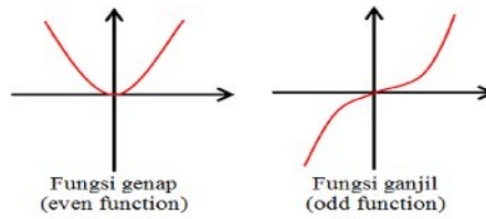
Gambar 1. Fungsi ganjil dan genap.
