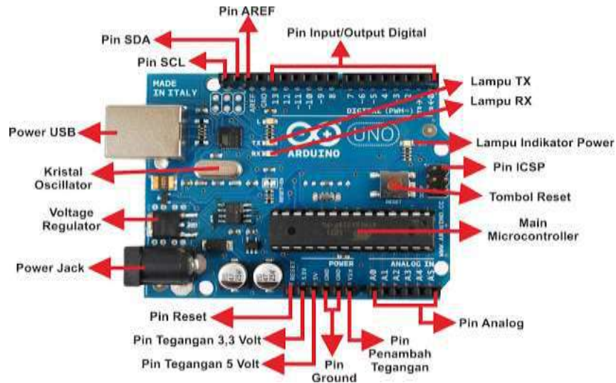
Gambar 2.1. Microkontroller Arduino UNO
