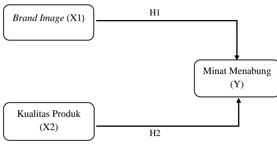
Gambar 2. 1 Kerangka Berfikir
