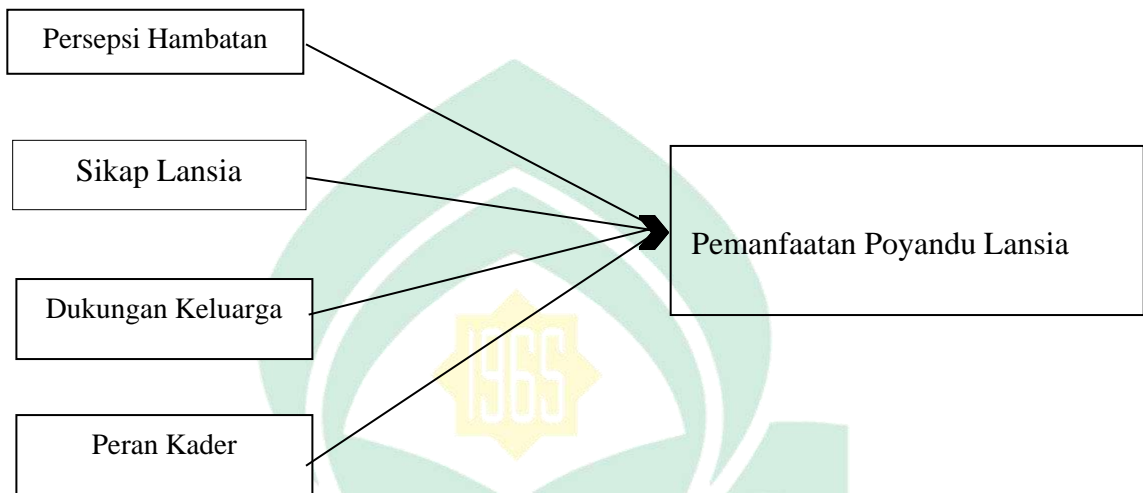
Gambar 3.2 Kerangka Konsep
