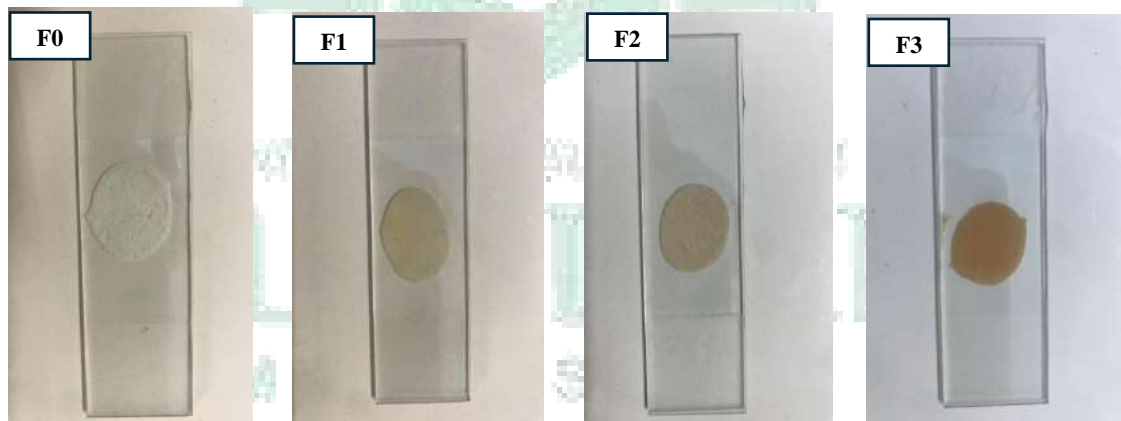
Gambar 30. Hasil Uji Homogenitas Krim Ekstrak Kulit Batang Kayu Jawa
