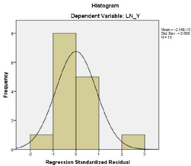
Gambar 4.1 Uji Normalitas
