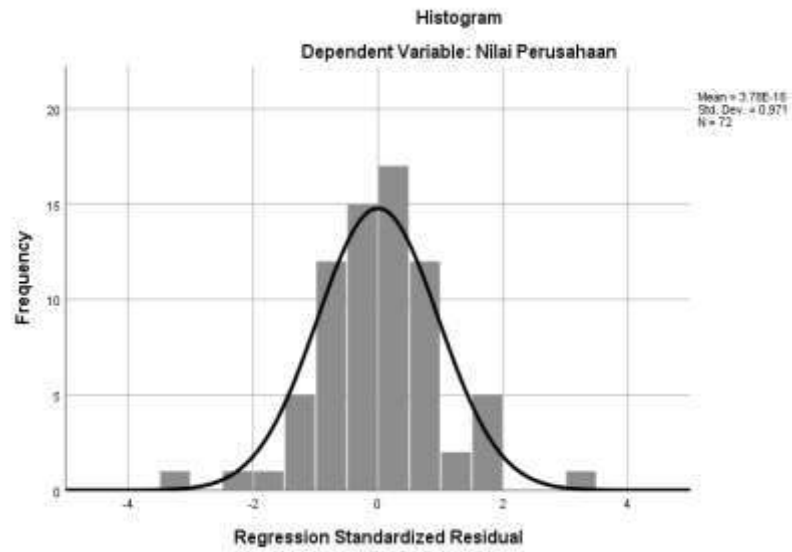
Gambar 4.1 Hasil Uji Normalitas-Grafik Histogram
