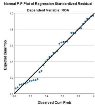
Gambar 4. 2 Uji Normalitas-Normal Probability Plot Persamaan I
