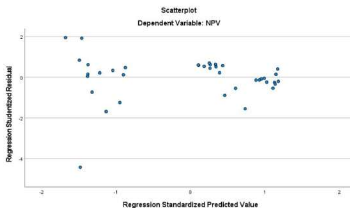
Gambar 4. 6 Uji Heteroskedastisitas-Scatterplot Persamaan II
