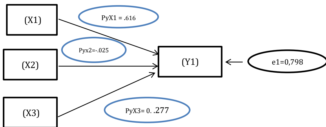
Gambar 4. 7 Model Path Analysis (Analisis Jalur) persamaan I
