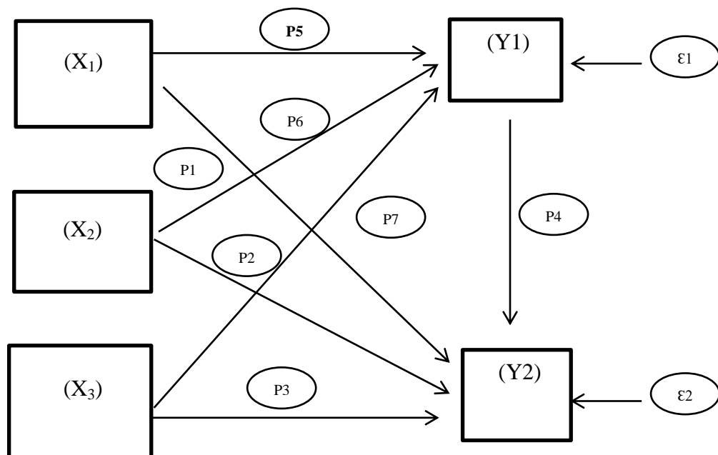
Gambar 3. 1 Kerangka Jalur (Path)
