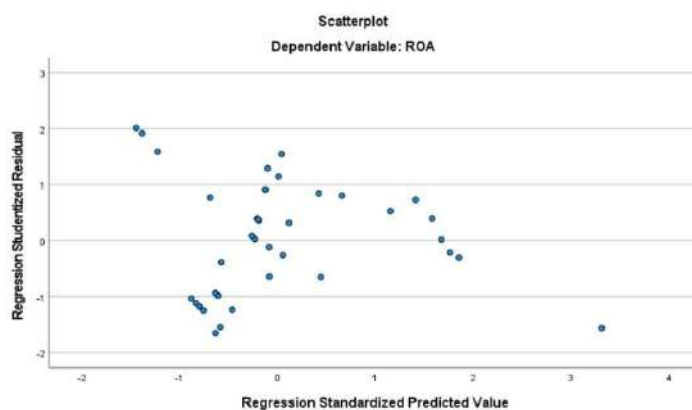
Gambar 4. 5 Uji Heteroskedastisitas-Scatterplot Persamaan I
