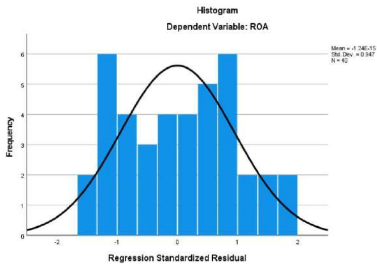
Gambar 4. 1 Uji Normalitas-Grafik Histogram Normal Persamaan I
