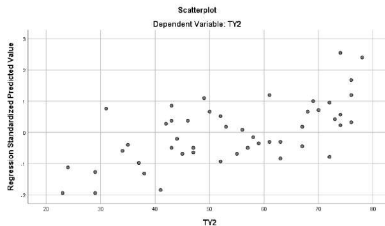
Gambar 4.2 Hasil Uji Heteroskedastisitas Program Guru Asuh terhadap Motivasi Belajar
