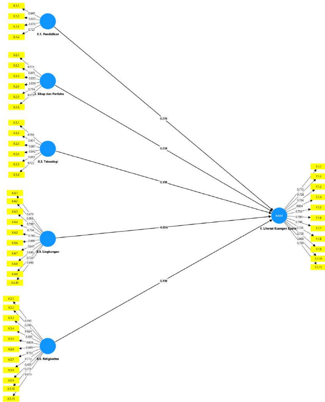
Gambar 4.1. Model Uji Tahap Awal (Outer Loading)
