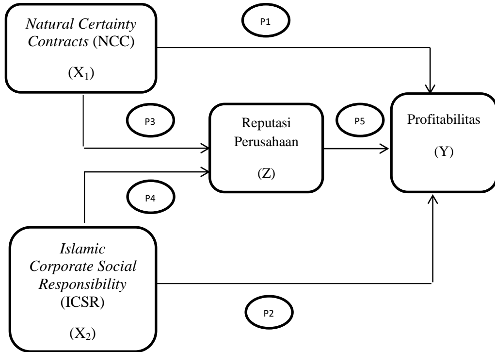
Gambar 3. 1 Kerangka Jalur ( Path )
