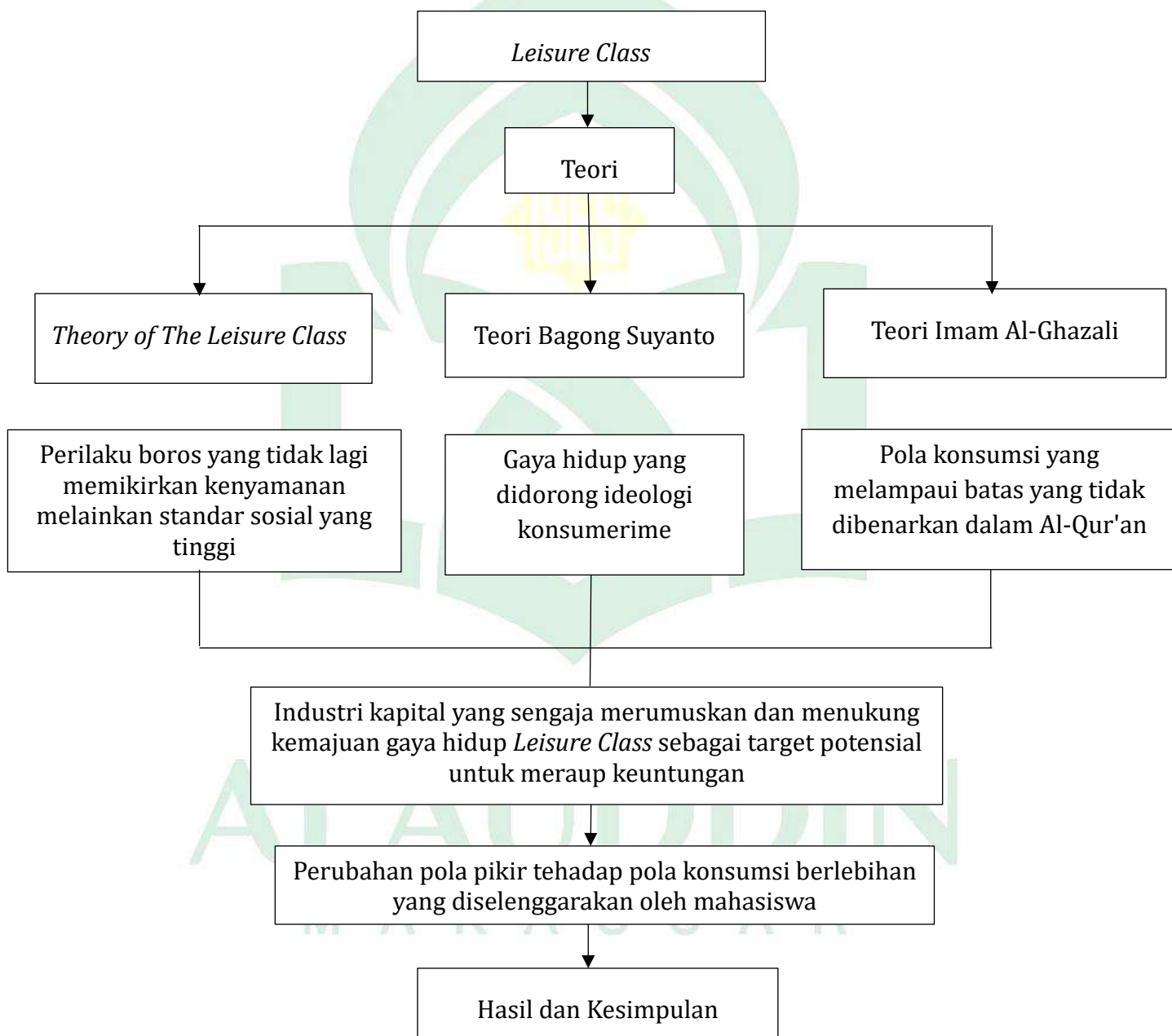
Gambar 2.1 Kerangka Teori
