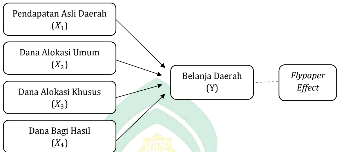
Gambar 2. 1 Kerangka Pikir
