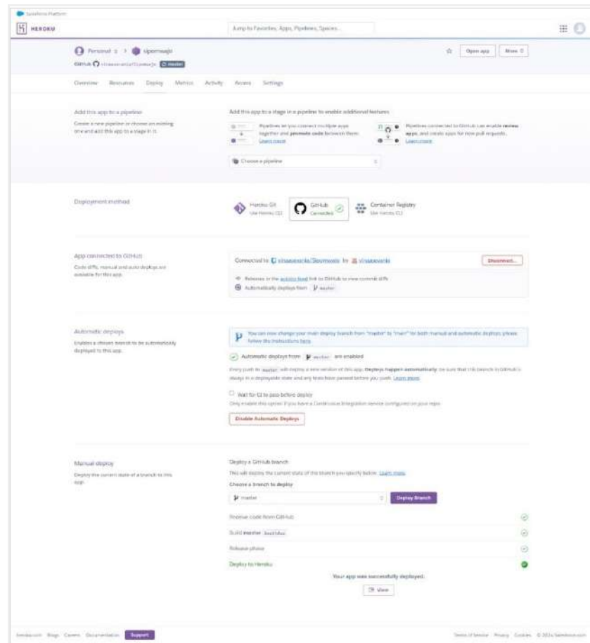
Gambar V. 4 Konfig Github
