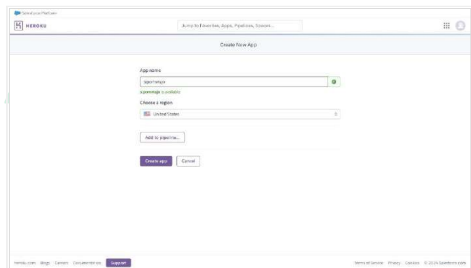
Gambar V. 1 Pembuatan Aplikasi
