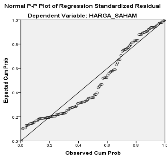
Gambar 4.5 Uji Normalitas
