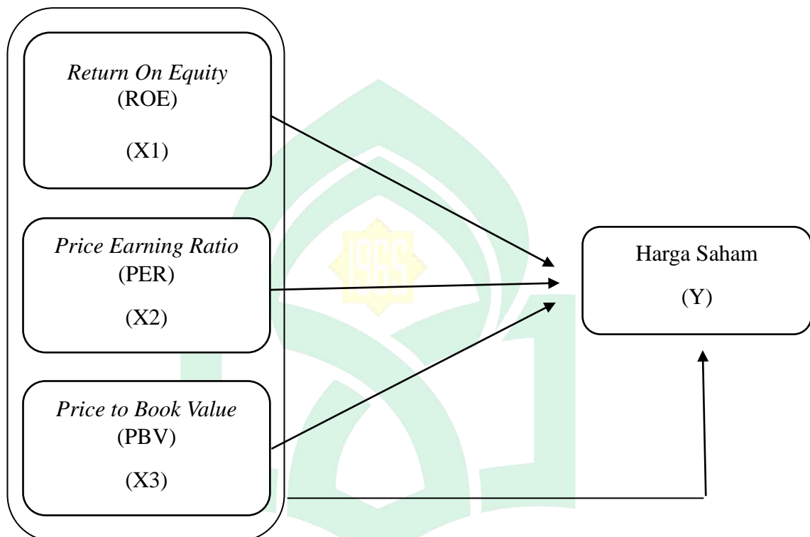
Gambar 2.1 Kerangka Berpikir
