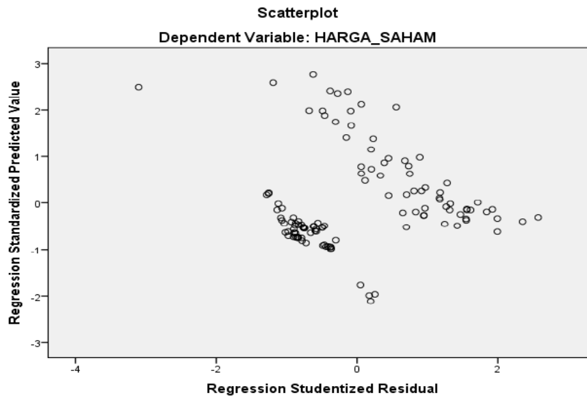
Gambar 4.6 Grafik Scatterplot
