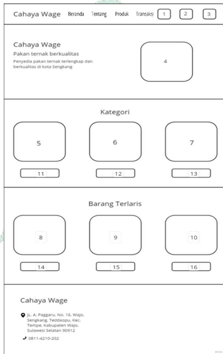
Gambar III. 11 Desain Antarmuka Menu Beranda
