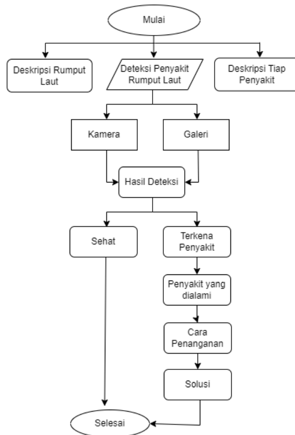
Gambar IV. 3 Alur sistem yang sedang diusulkan
