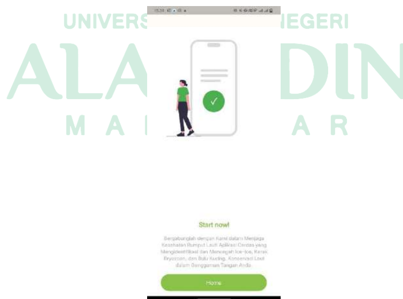
Gambar V. 3 Antarmuka Mulai
