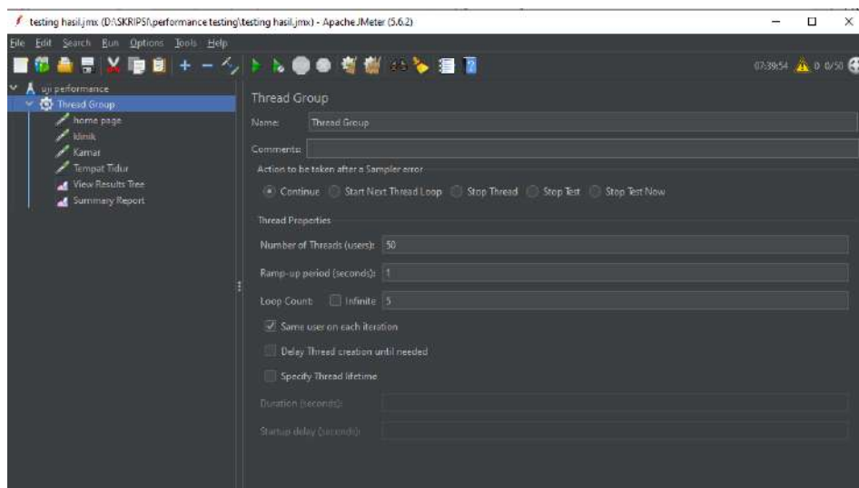
Gambar V.15 Skenario Pengujian Beban Berat
