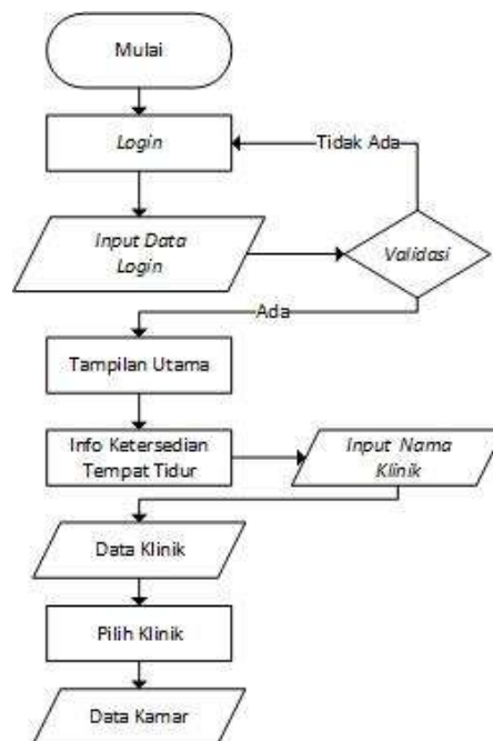
Gambar IV.1 Flowchart Pada Mobile JKN
