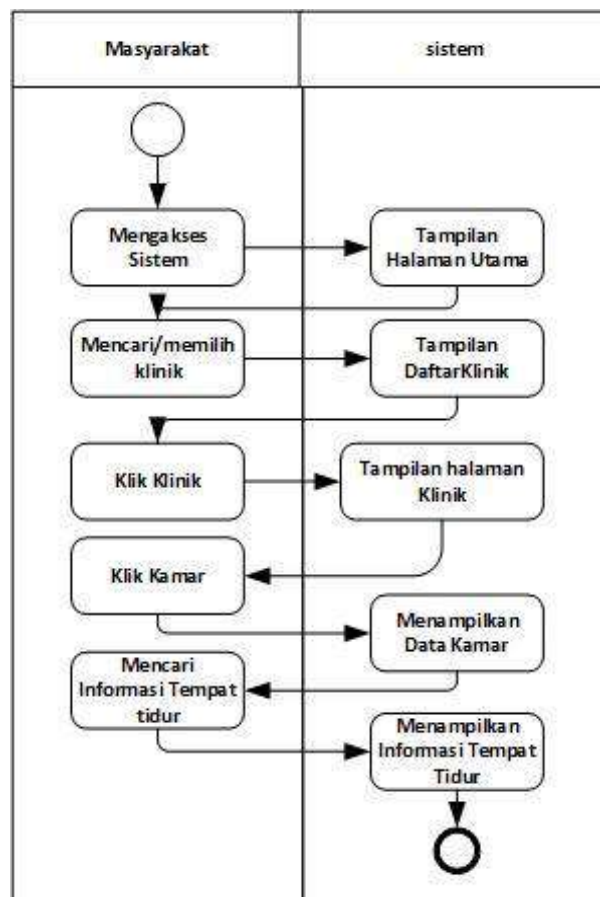
Gambar IV.15 Activity Diagram Pada Fitur Informasi Tempat Tidur
