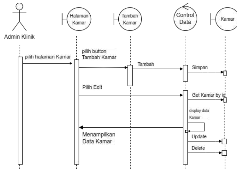
Gambar IV. 11 Sequence Diagram Tambah Tempat Tidur
