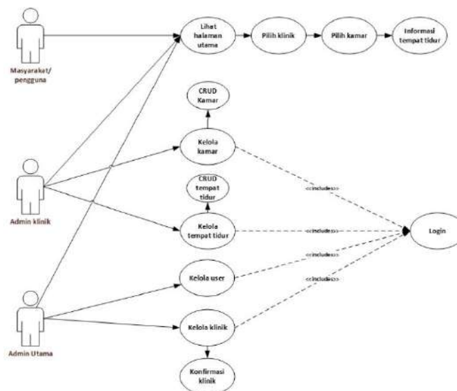
Gambar IV.6 Use Case Diagram yang Diusulkan
