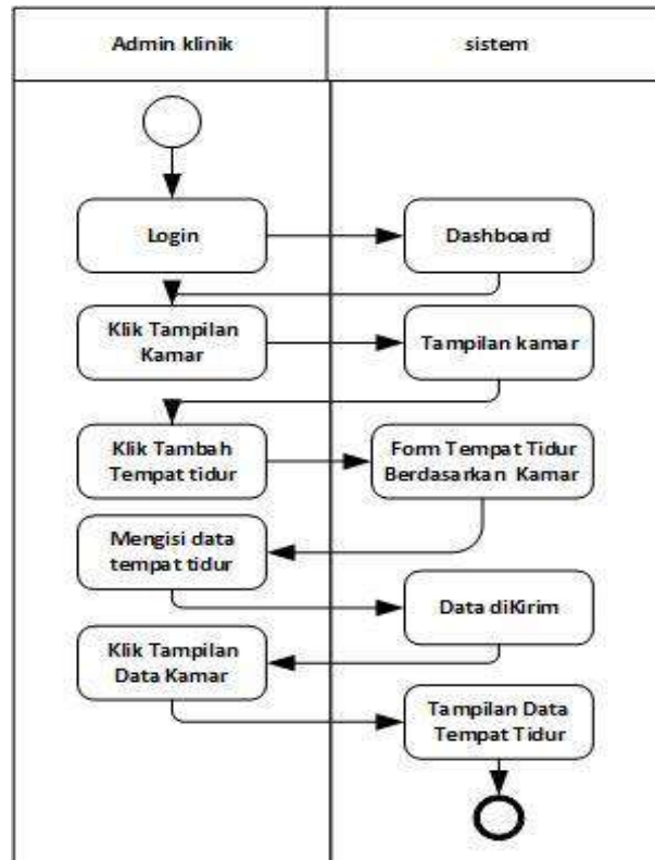
Gambar IV.14 Activity Diagram Pada Fitur Olah Data Tempat Tidur
