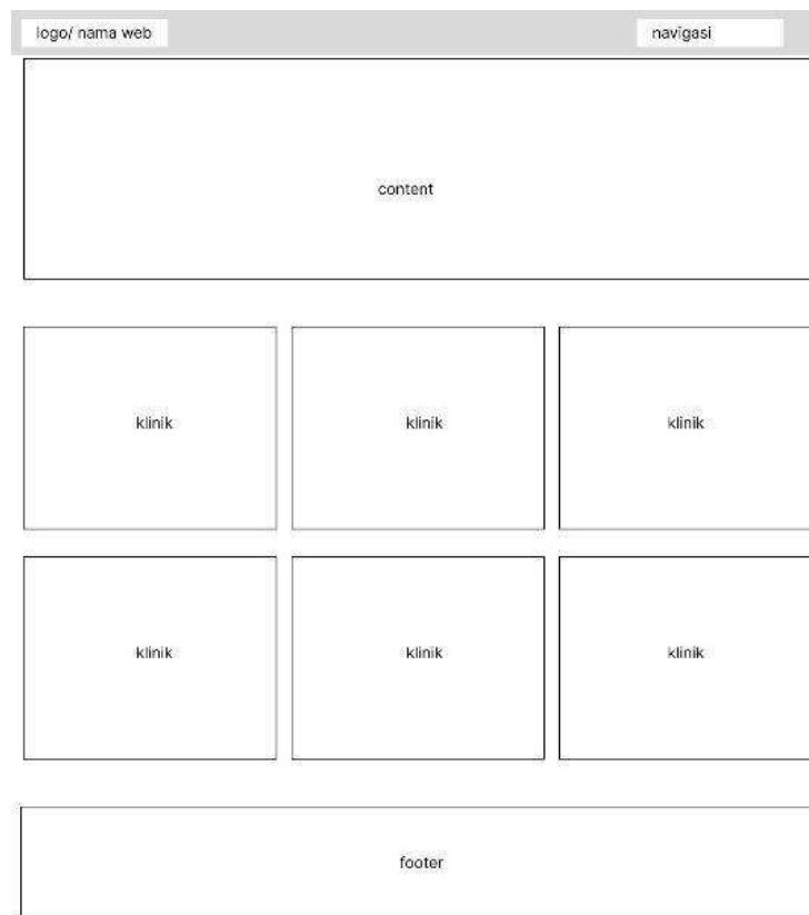
Gambar IV.29 Wireframe Menu Klinik
