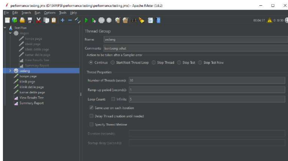
Gambar V.14 Skenario Pengujian Beban Sedang
