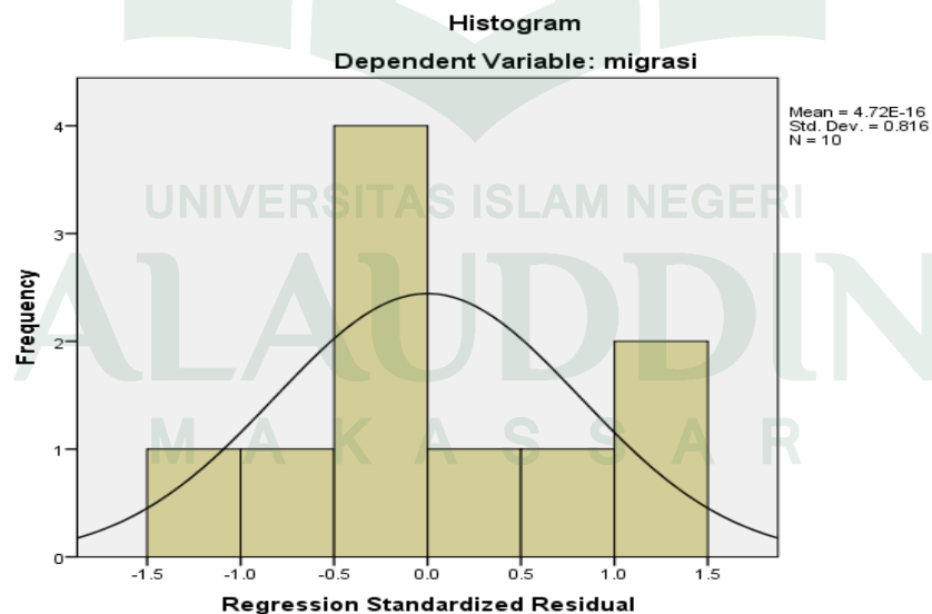
Gambar 4.1 Grafik Histogram
