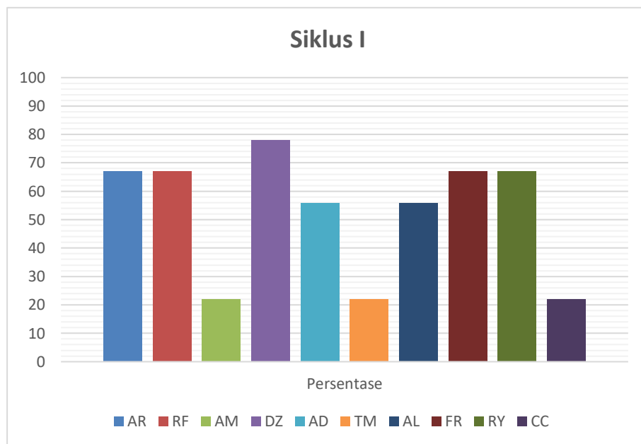
Gambar 4. 1 Diagram Batang Perkembangan Kemampuan Mengenal Angka Anak pada Siklus I
