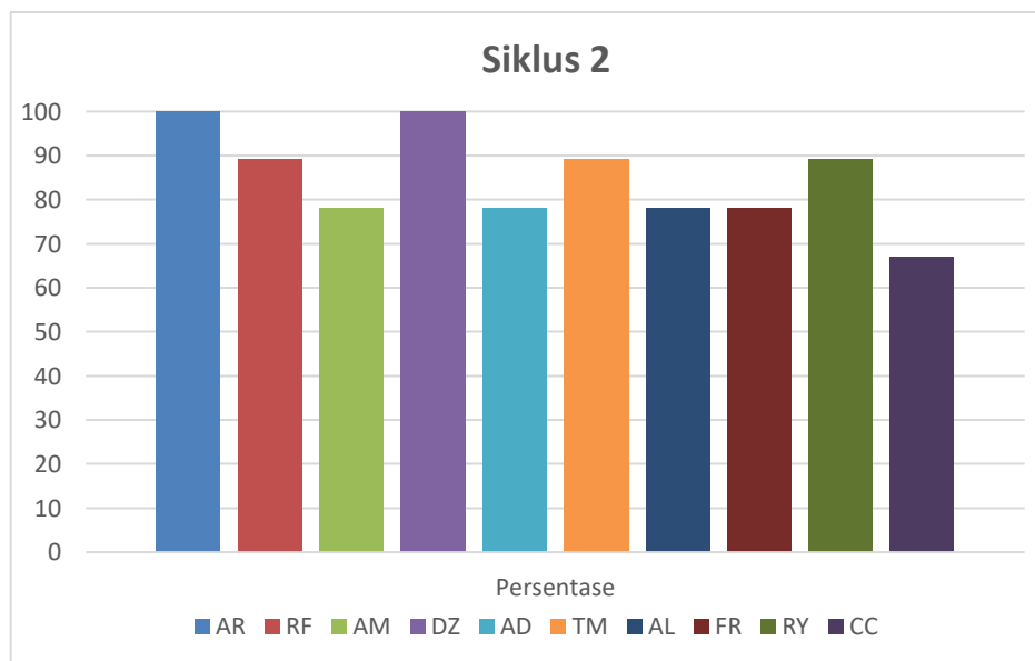
Gambar 4. 2 Diagram Batang Perkembangan Kemampuan Mengenal Angka Anak pada Siklus II
