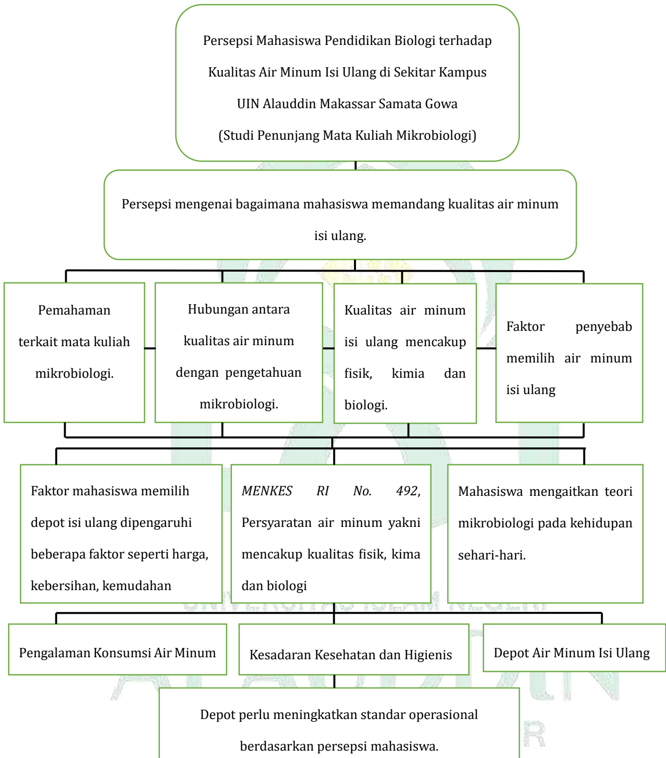
Gambar 2. 2 Kerangka Konseptual
