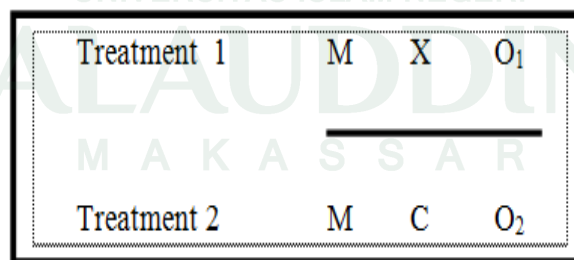
Gambar 3.1 Desain Penelitian
