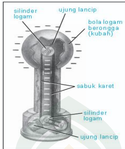
Gambar 2.4: Generator Van De Graaff
