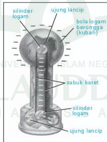
Gambar 5 : Generator Van de Graaff
