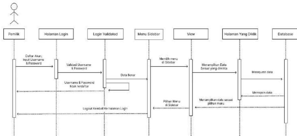
Gambar IV. 6 Sequence Diagram (Pemilik Villa)
