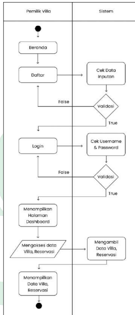
Gambar IV. 9 Activity Diagram Pemilik Villa
