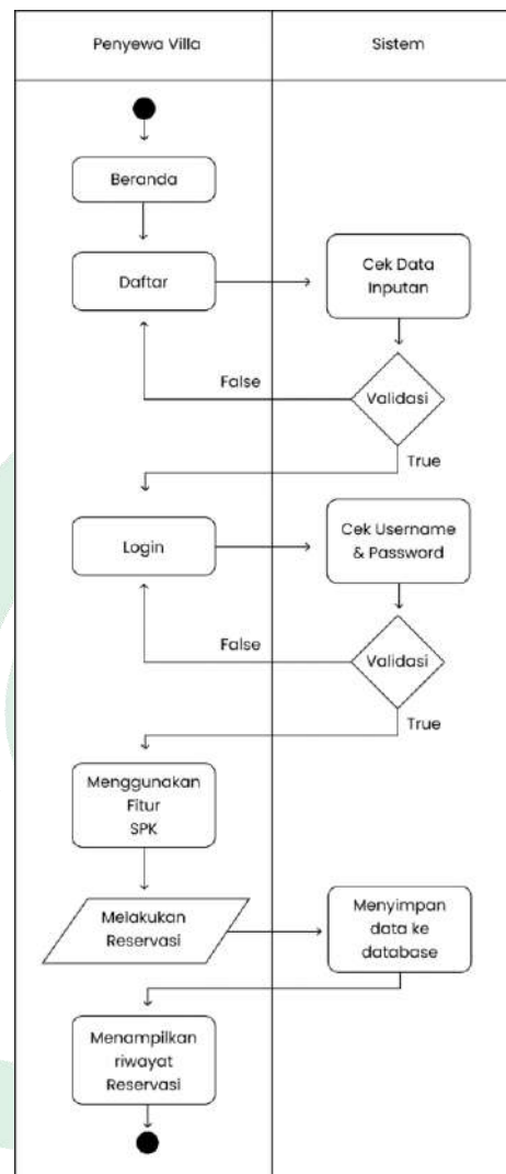
Gambar IV. 10 Activity Diagram Penyewa Villa
