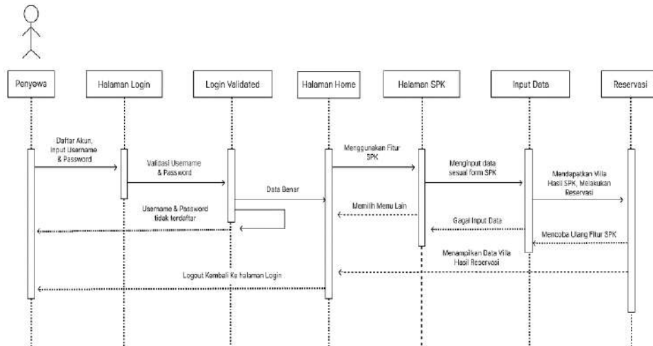
Gambar IV. 7 Sequence Diagram (Penyewa)
