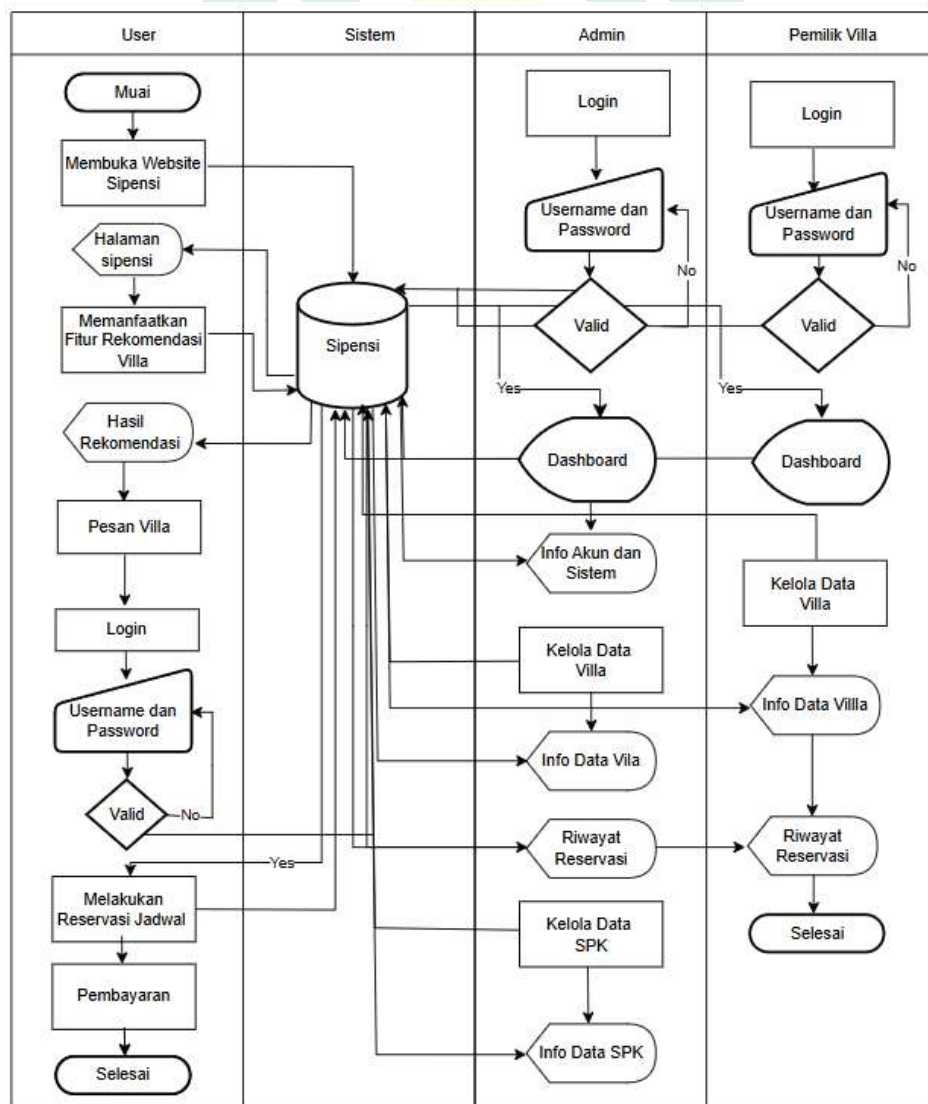
Gambar IV. 2 Flowchart Alur sistem yang diusulkan
