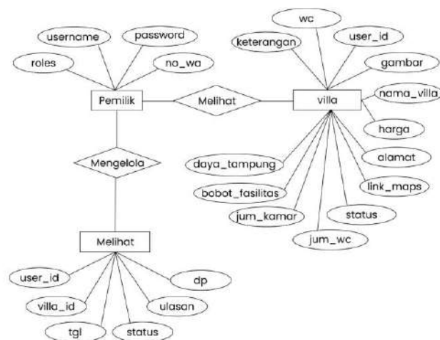
Gambar IV. 12 ERD ( Entity Relationship Diagram Pemilik Villa )
