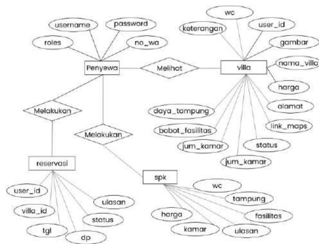
Gambar IV. 13 ERD ( Entity Relationship Diagram Penyewa)
