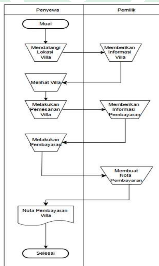
Gambar IV. 1 Flowchart Sistem yang sedang berjalan
