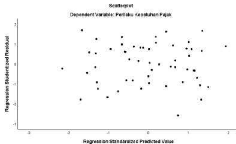
Gambar 4. 2 Hasil Uji Heteroskedastisitas – Grafik ScatterPlot
