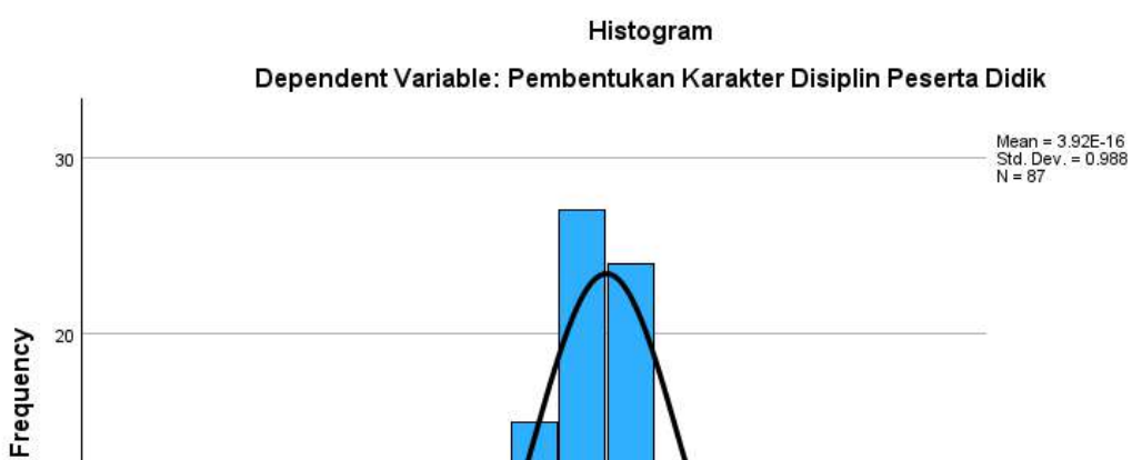
Gambar 4. 1 Histogram Uji Normalitas
