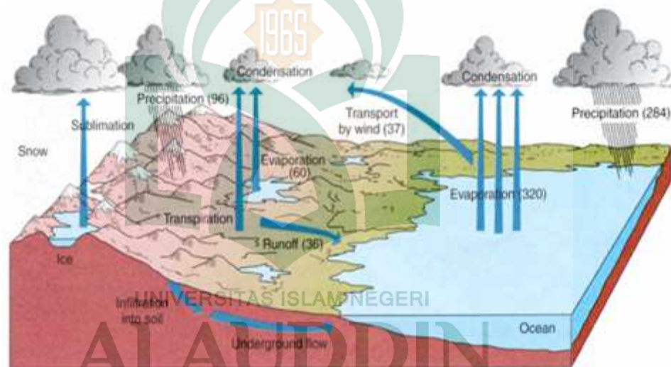
Gambar 2.1 Siklus Hidrologi
