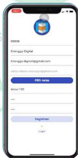
Gambar 2.2 Daftar Akun
