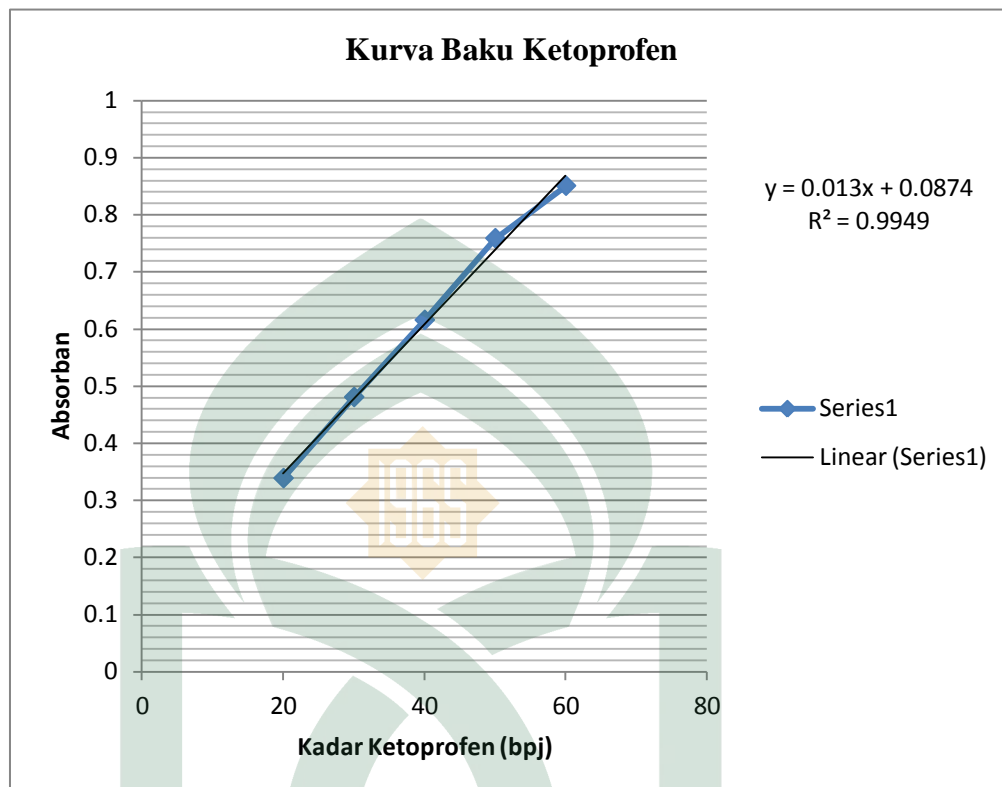
Gambar 3. Grafik Kurva Baku Ketoprofen
