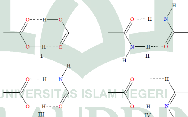
Gambar 1. Ikatan hidrogen dalam kokristal ((Issa, 2011: 34; 90)
