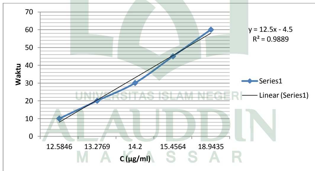
Gambar 5. Kurva Hasil Disolusi Ketoprofen
