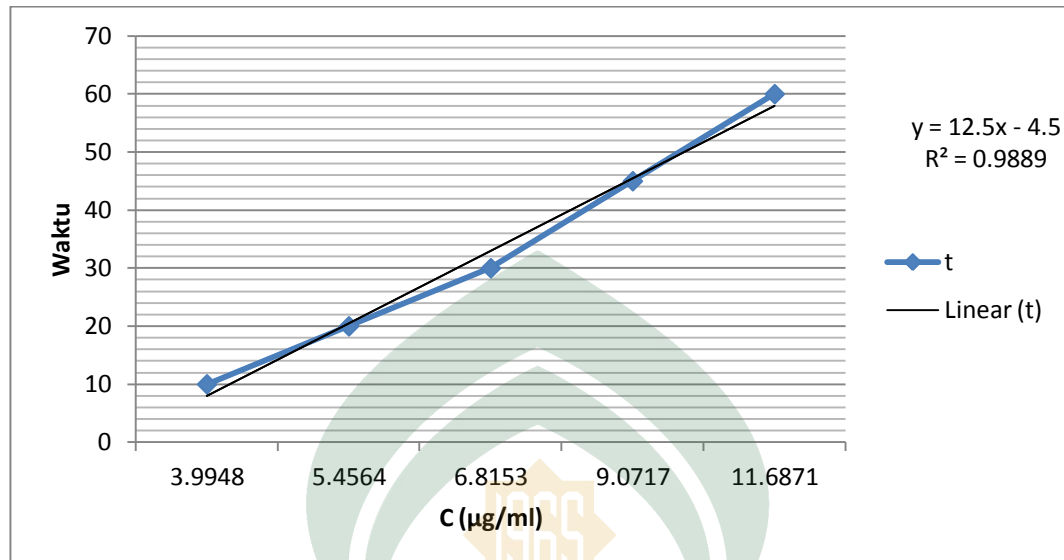
Gambar 4. Kurva Hasil Disolusi Kokristal Ketoprofen
