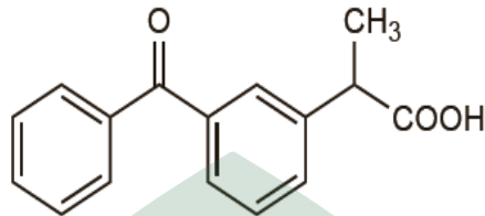
Gambar 2. Struktur Ketoprofen (Sweetman, 2009: 73).
