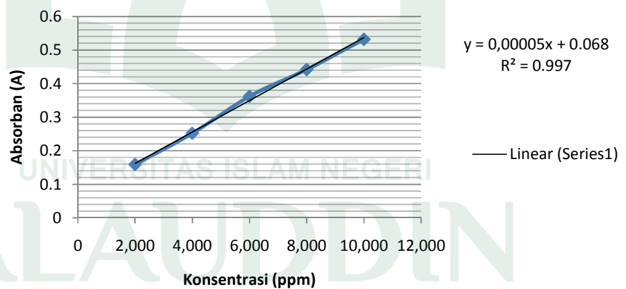
Gambar 1. Kurva baku Natrium Benzoat pada panjang gelombang 288 nm.
