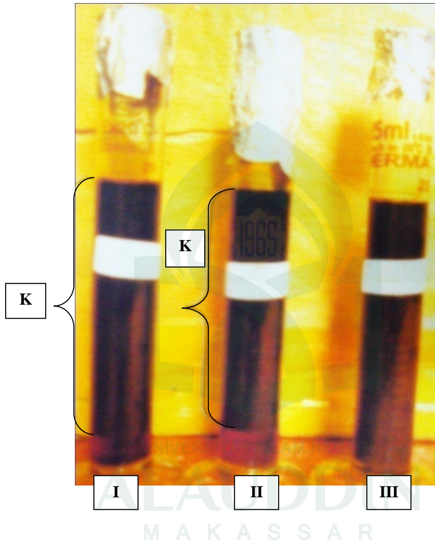
Gambar 16. Foto Uji Volume Kriming Pada Krim Dengan Kombinasi Emulgator Tween 60 Dan Span 60 Pada Kondisi Setelah Penyimpanan Dipercepat
