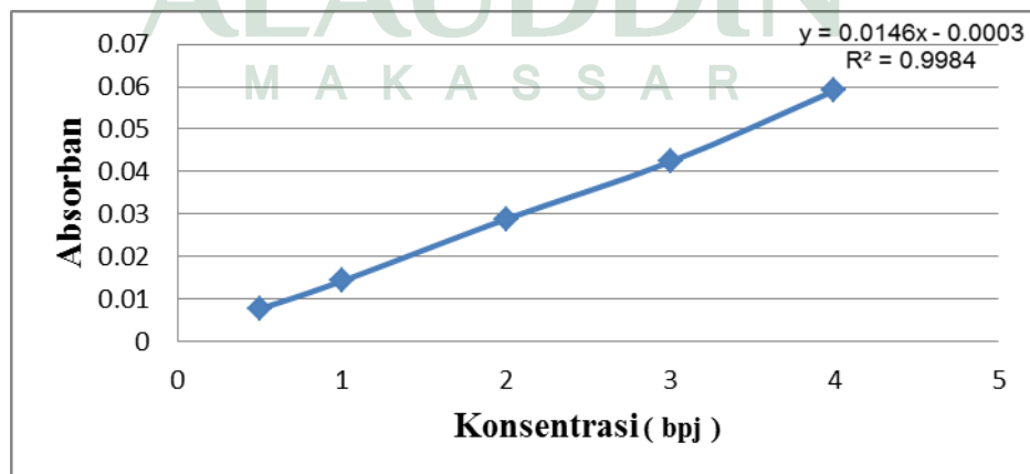
Gambar 3 : Kurva baku besi (Fe)
