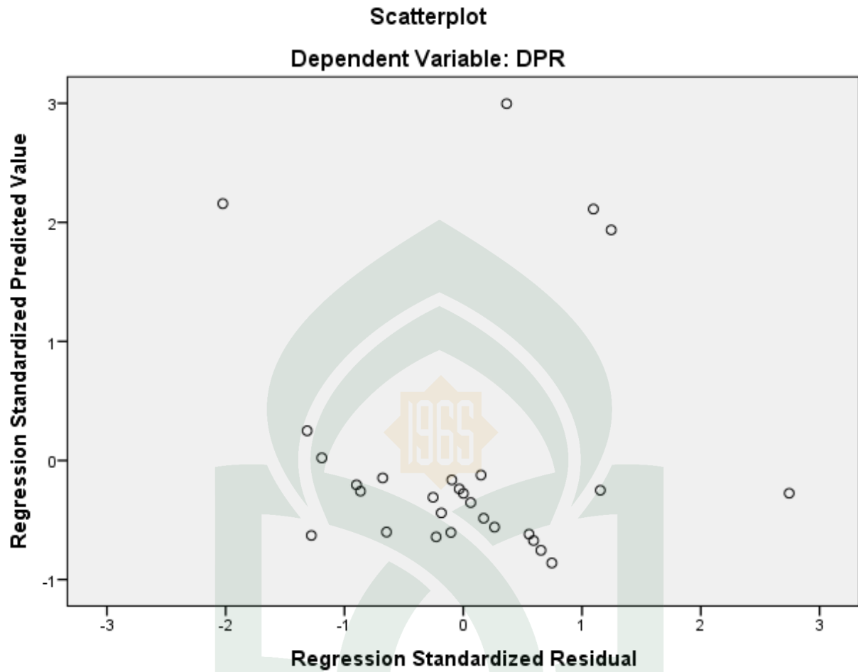
Gambar 4.3 Grafik scatterplot
