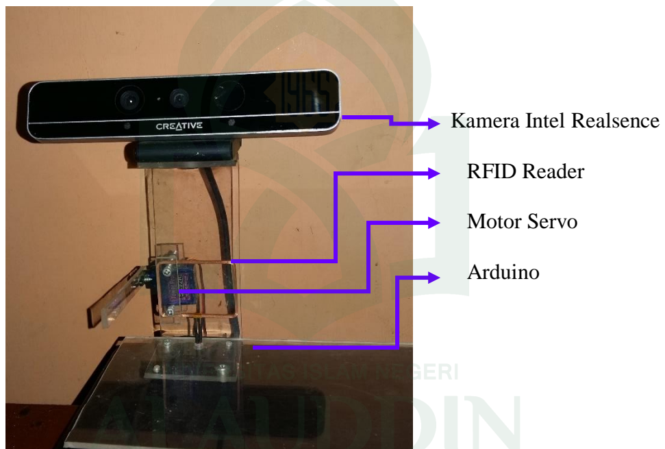
Gambar V- 1. Hasil Miniatur Sistem Parkir Otomatis
