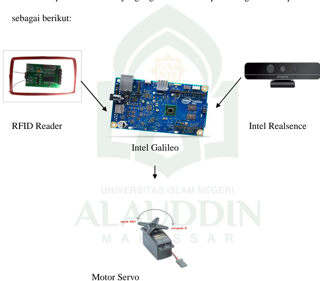
Gambar IV- 2. Susunan alat yang digunakan
