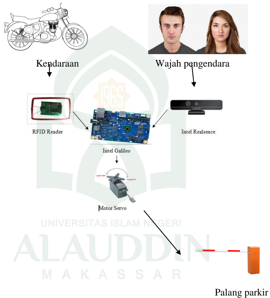
Gambar IV- 3. Desain Keseluruhan Alat
