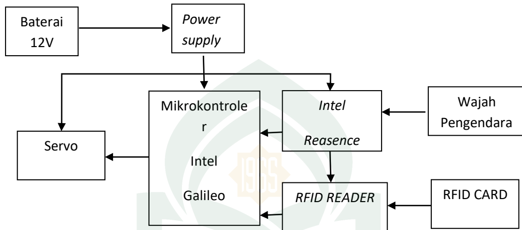
Gambar IV- 1. Diagram Blok Sistem Alat
