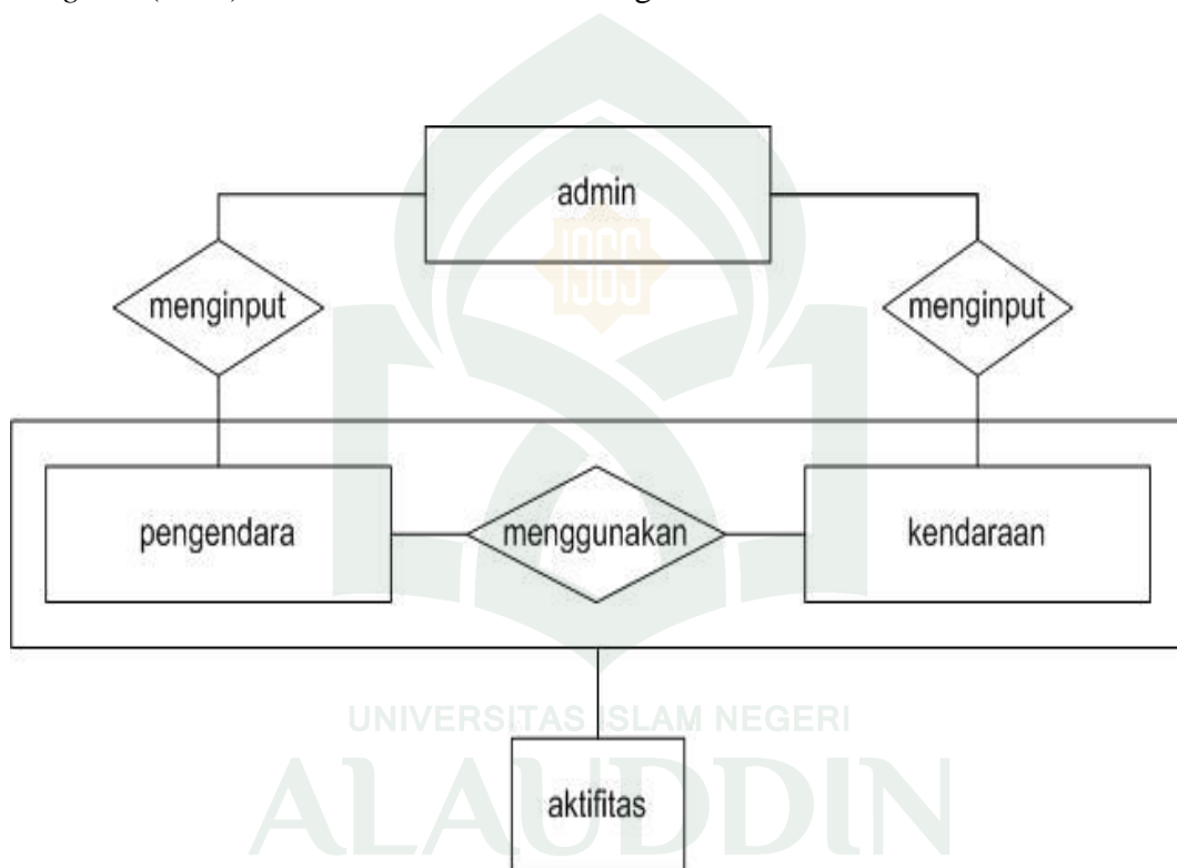
Gambar IV- 7. Rancangan ERD
