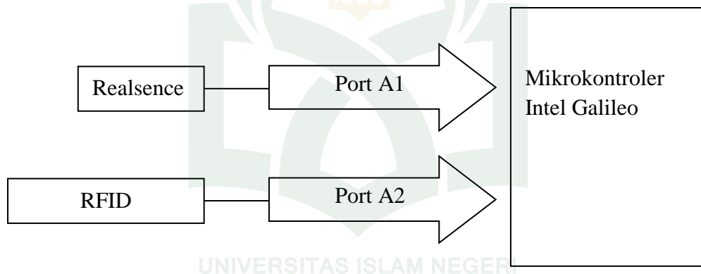
Gambar IV- 4. Rancangan Realsence dan RFID
