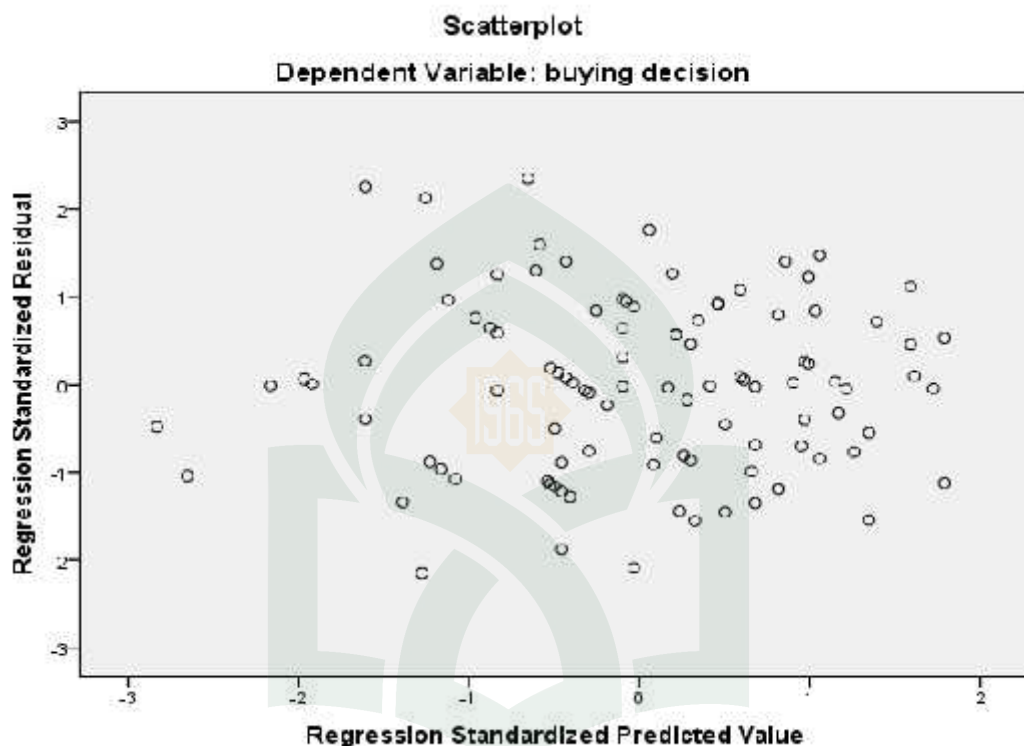
Gambar 4.2 Uji Heterokedastisitas
