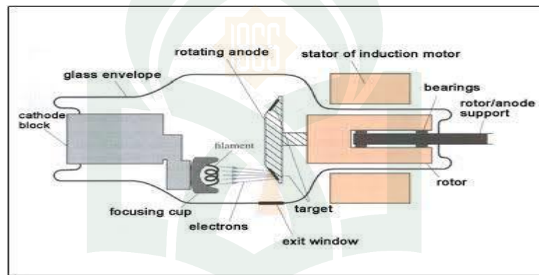
Gambar 2.5 Tabung pesawat sinar X (Sumber: http://www.google.image.com )
