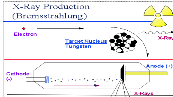
Gambar 2.6 Produksi sinar-X Bremsstrahlung (Sumber: Http://www.google.image.com )
