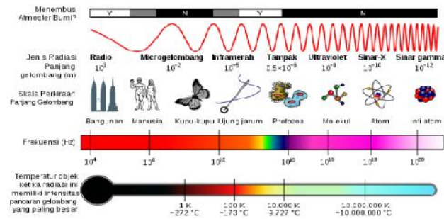
Gambar 2.1. Spektrum Gelombang Elektromagnetik (Sumber: Arif, 2015)
