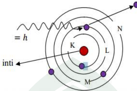
Gambar 2.2 Proses efek fotolistrik (Sumber:Gusmavita, 2011)
