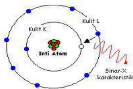
Gambar 2.7 Ilustrasi terjadinya sinar-X karakteristik (Sumber: http://www.google.image.com )
